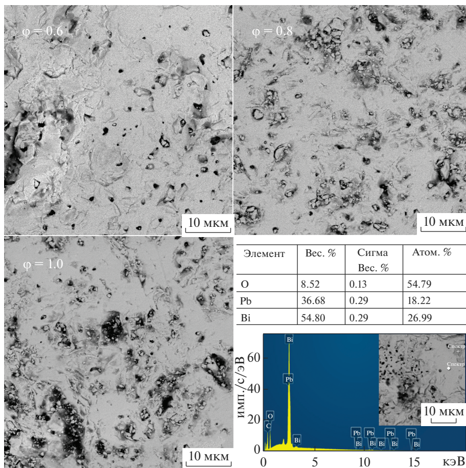
Рис. 2. Микрофотографии образцов \phi - \text{Bi}_8\text{Pb}_5\text{O}_{17} , синтезированных пиролизом маннит-нитратных композиций, с различным соотношением окислителя и восстановителя \phi = 0.6; 0.8; 1 в режиме “фазового контраста” и пример микрозондового анализа участка керамики с погрешностью химического состава, определенной по измерениям в разных точках.
