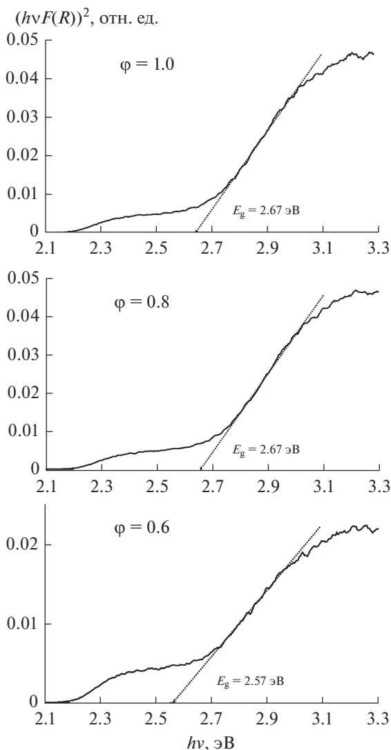
Рис. 3. Аппроксимация спектров оптического поглощения в предположении модели прямых разрешенных переходов для образцов \phi -Bi 8 Pb 5 O 17 , синтезированных пиролизом маннит-нитратных композиций, с различным соотношением окислителя и восстановителя \phi = 0.6; 0.8; 1 .
