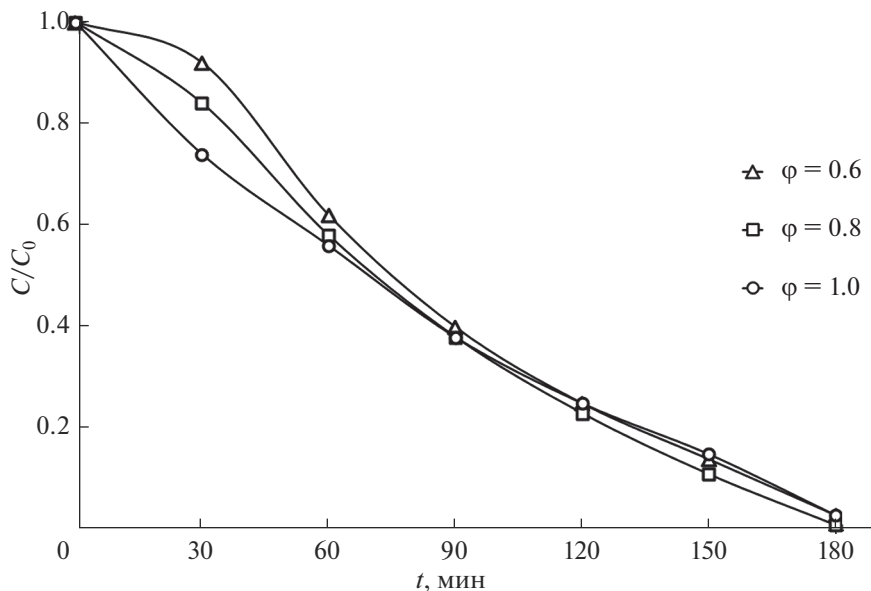
Рис. 4. Фотокаталитическая деградация красителя МО под воздействием облучения на образцах \phi\text{-Bi}_8\text{Pb}_5\text{O}_{17} , синтезированных пиролизом маннит-нитратных композиций, с различным соотношением окислителя и восстановителя \phi = 0.6; 0.8; 1 .
