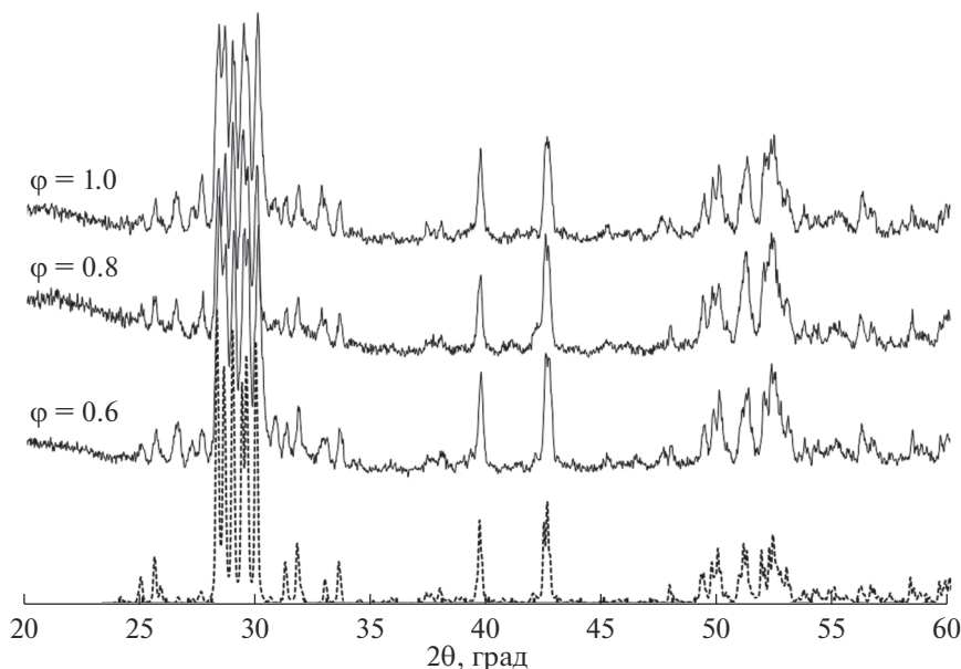
Рис. 1. Дифрактограммы образцов \varphi - \text{Bi}_8\text{Pb}_5\text{O}_{17} , синтезированных пиролизом маннит-нитратных композиций, с различным соотношением окислителя и восстановителя \varphi = 0.6; 0.8; 1 после 30 ч при 560^\circ\text{C} (сплошная линия) и расчетная дифрактограмма \varphi - \text{Bi}_8\text{Pb}_5\text{O}_{17} по карточке COD № 96-152-6076 (пунктирная линия).
