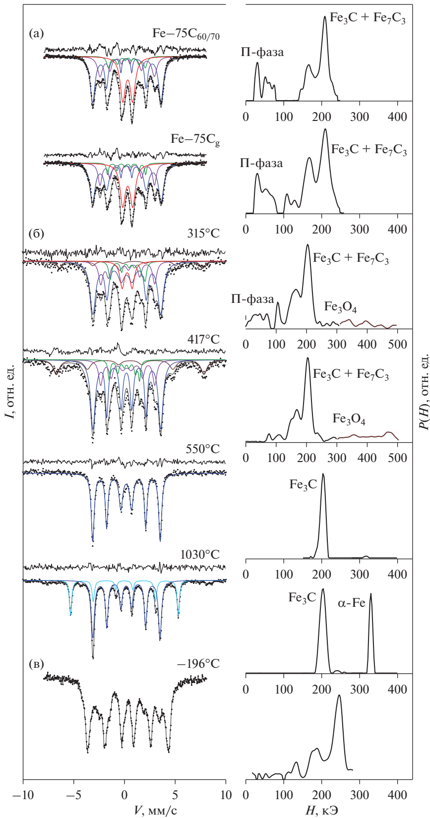
Рис. 2. Мёссбауэровские спектры и функции распределения сверхтонких магнитных полей: а – образцов Fe–75C 60/70 и Fe–75C g после 8 ч МС; б – композита Fe 3 C/Fe 7 C 3 /П-фаза/C ам после нагрева до различных температур; в – композита Fe 3 C/Fe 7 C 3 /П-фаза/C ам при температуре жидкого азота.
