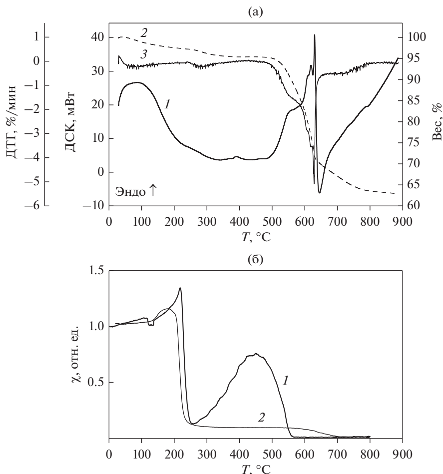
Рис. 4. Кривые ДСК (1), ТГ (2) и ДТГ (3) композита \text{Fe}_3\text{C}/\text{Fe}_7\text{C}_3/\Pi\text{-фаза}/\text{C}_{\text{ам}} (а) и кривые температурной зависимости магнитной восприимчивости (б) при нагреве (1) и охлаждении (2) [17].
