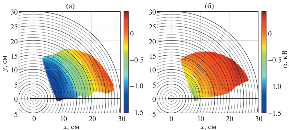
Рис. 6. Двумерные распределения электрического потенциала плазмы по данным ЗПТИ на токамаке Т-10 для режима B_t = 2.2 \text{ Тл} , I_{pl} = 230 \text{ кА} , \bar{n}_e \approx (1.1 \pm 0.1) \times 10^{19} \text{ м}^{-3} : для омического режима (а); для режима с нецентральной ЭЦР-нагревом (б). Штриховой линией обозначены эквипотенциальные линии; цветом – значение потенциала плазмы.
