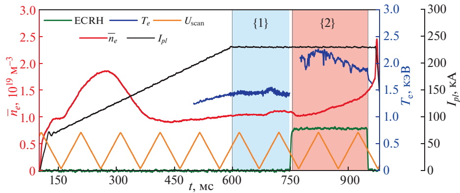
Рис. 1. Сценарий типичного исследуемого разряда #73203 ( B_t = 2.2 Тл, I_{pl} = 230 кА): красная линия – среднехордовая электронная плотность (левая шкала); синяя – электронная температура (правая шкала 1); черная – ток плазмы (правая шкала 2); зеленая – индикация ЭЦР-нагрева; оранжевая – сканирующее напряжение на отклоняющих пластинах с периодом 100 мс и амплитудой от -7.6 до -2.3 кВ (шкала для величины U_{scan} не приводится); {1} – временной интервал стационарной омической стадии разряда; {2} – временной интервал стадии с нецентральной ЭЦР-нагревом мощностью P_{ECRH} = 1.7 МВт ( r = 15 см).
