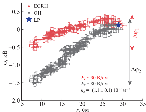
Рис. 4. Профили электрического потенциала плазмы с фиксированной среднехордовой электронной плотностью \bar{n}_e = (1.1 \pm 0.1) \times 10^{19} \text{ м}^{-3} . Красные точки – профиль с нецентральной ЭЦР-нагревом; серые – профиль с омическим нагревом. На периферии (синей звездой) приведено измерение с помощью зонда Ленгмюра (LP). Стрелками указаны \Delta\phi_1 , \Delta\phi_2 – диапазоны обоих профилей потенциала. Погрешность измерения электрического потенциала плазмы \Delta\phi \approx \pm 0.1 \text{ кВ} , пространственное разрешение \Delta r \approx \pm 1 \text{ см} .
