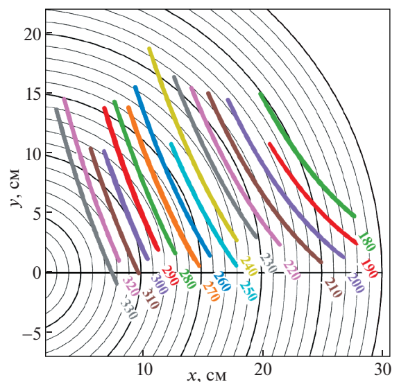
Рис. 3. Область измерения ЗПТИ для режима Т-10 с магнитным полем на оси B_t = 2.2 Тл, током плазмы I_{pl} = 230 кА. Цветом показаны детекторные линии, рассчитанные для значений энергии зондирующего пучка E_{beam} = 180\text{--}330 кэВ.
