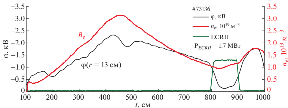
Рис. 5. Временная эволюция среднехордовой электронной плотности, электрического потенциала плазмы на r = 13 \text{ см} в импульсе #73136 ( B_t = 2.2 \text{ Тл} , I_{pl} = 230 \text{ кА} ): черная линия – потенциал плазмы (левая шкала); красная – плотность плазмы (правая шкала); зеленая – индикация ЭЦР-нагрева. Вертикальная ось для потенциала направлена в сторону отрицательных значений.
