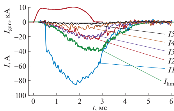
Рис. 2. Подборка типичных сигналов, характеризующих работу систем питания внутрикамерных электродов. Ток плазменной пушки приведен в качестве масштаба по времени, радиальные сегменты плазмодриемника пронумерованы от центра к краю 11–15. Токи плазменной пушки I_{\text{gun}} и лимитеров I_{\text{lim}} для наглядности показаны с обратной полярностью.
