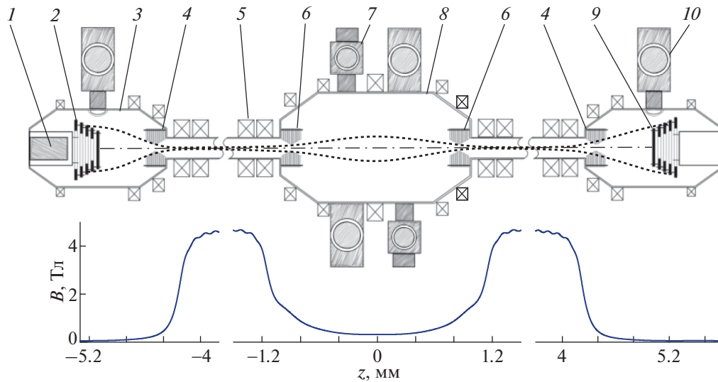
Рис. 1. Схема расположения внутрикамерных электродов в установке ГОЛ-NB (вид сверху) и профиль магнитной индукции вдоль оси: 1 – плазменная пушка, 2 – входной радиально-секционированный плазмодриемник, 3 – бак расширителя, 4 – лимитерные сборки в расширителях, 5 – катушка секции сильного поля, 6 – лимитерные сборки в центральной ловушке, 7 – инжектор быстрых атомов водорода, 8 – центральная ловушка, 9 – выходной радиально-секционированный плазмодриемник, 10 – модуль системы откачки. Пунктирной линией условно обозначена силовая линия, касающаяся внутренней апертуры всех лимитеров. Секции сильного поля, состоящие из 28 катушек каждая, показаны частично.
