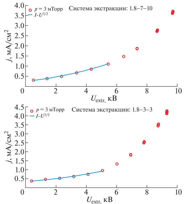
Рис. 5. Зависимость плотности тока отрицательных ионов на цилиндр Фарадея от напряжения экстракции для систем экстракции: а) 1.8–7–10; б) 1.8–3–3 при падающей СВЧ-мощности P_{\text{гвр}} = 4.9 \text{ кВт} . В области малых напряжений построена аппроксимация I \sim U^{3/2} .
