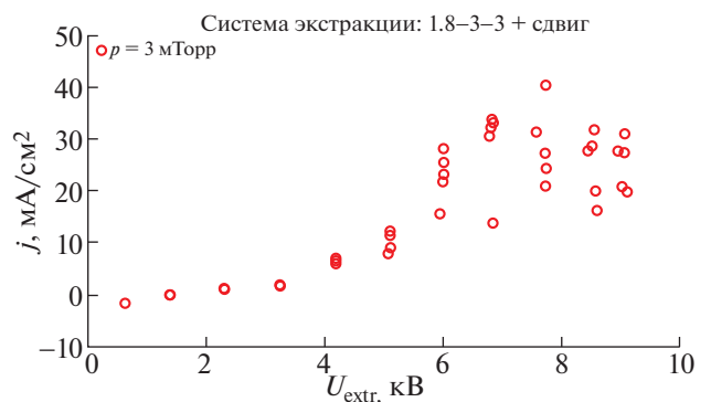
Рис. 6. Зависимость плотности тока отрицательных ионов на цилиндр Фарадея от напряжения экстракции для сдвинутой системы экстракции 1.8–3–3 при падающей СВЧ-мощности P_{\text{гвр}} = 4.9 \text{ кВт} .
