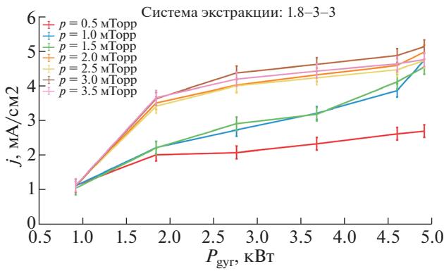
Рис. 4. Зависимость плотности тока отрицательных ионов водорода на цилиндр Фарадея от мощности падающего СВЧ-излучения при различных значениях давления нейтрального газа для системы экстракции 1.8–3–3.
