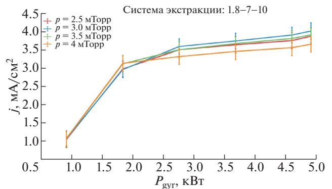
Рис. 3. Зависимость плотности тока отрицательных ионов водорода на цилиндр Фарадея от мощности падающего СВЧ-излучения при различных значениях давления нейтрального газа для системы экстракции 1.8–7–10.
