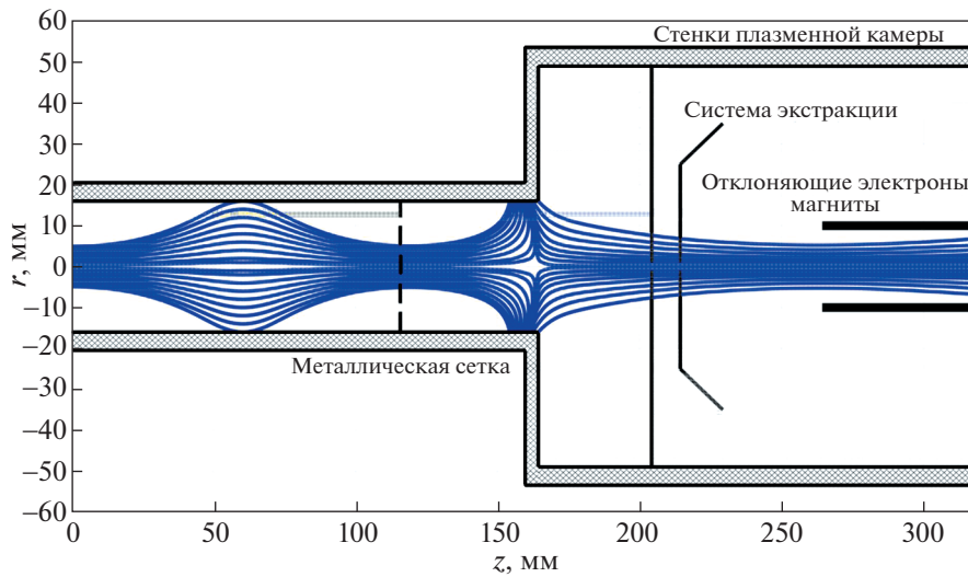
Рис. 2. Структура силовых линий магнитного поля экспериментальной установки.
