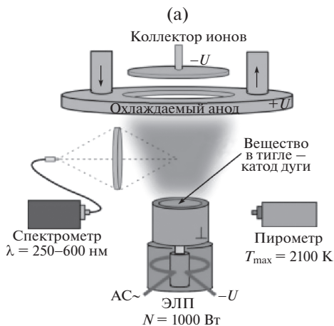
Рис. 8. а) – Схема дугового разряда с подогреваемым расходоуемым катодом; б) – зависимость интенсивности спектральных линий атомов и ионов гадолиния, а также средний заряд частиц за анодом как функция напряжения разряда [51].
