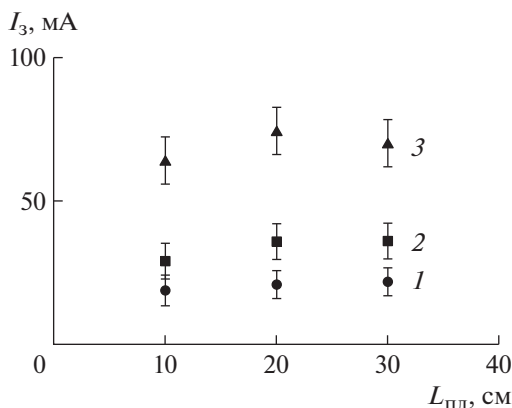
Рис. 8. Зависимость зондового тока в области ионного насыщения ( U = -150 В) от длины плазмы для трех значений тока разряда: 5 А (1), 9 А (2) и 20 А (3).
