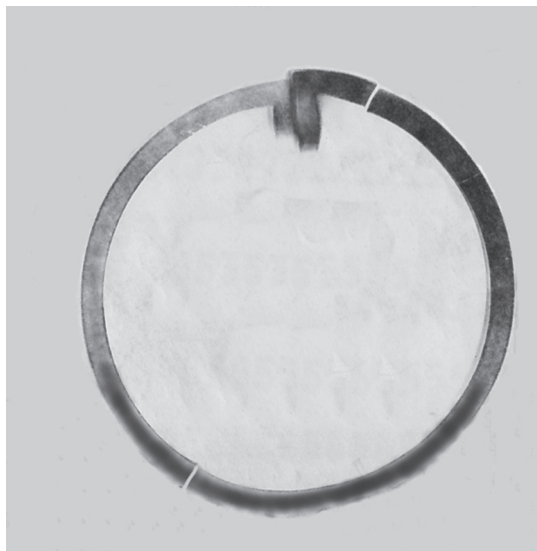
Рис. 2. Отпечаток электронного пучка, создаваемого кольцевым ленточным катодом, на термобумаге, закрепленной перпендикулярно оси волновода. Тонкая светлая линия, пересекающая в двух местах отпечаток термокатада, – тень от проволочного зонда.
