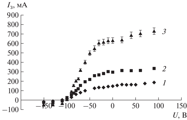
Рис. 4. Вольтамперные характеристики зонда для трех токов разряда: 5 А – 1, 9 А – 2, 20 А – 3. Длина плазмы 20 см. Горизонтальная погрешность меньше размера точки, вертикальная погрешность указана на графике 3. Для графиков 1 и 2 она пропорционально меньше.
