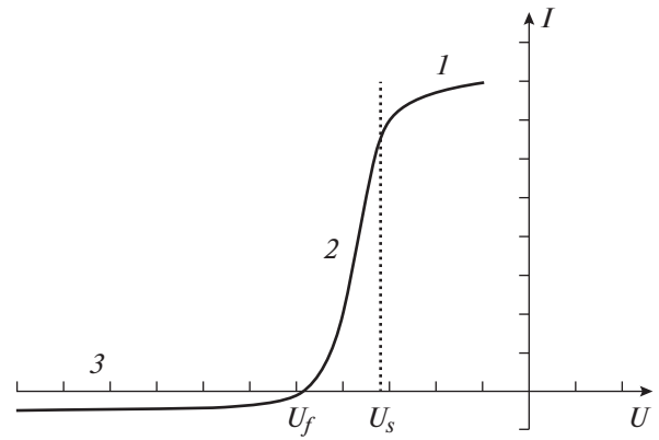
Рис. 5. Теоретическая ВАХ одиночного зонда: 1 – электронный ток насыщения, 2 – суммарный ток электронов и ионов, 3 – ионный ток насыщения; U_f – плавающий потенциал, U_s – потенциал пространства.
