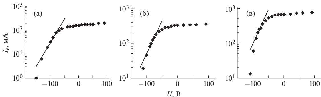
Рис. 6. Электронная ветвь ВАХ зонда в полулогарифмическом масштабе для трех токов разряда: 5 А (а), 9 А (б), 20 А (в). Прямая линия – аппроксимация графика в области ниже потенциала пространства. Длина плазмы 20 см.
