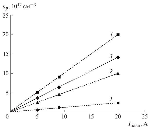
Рис. 10. Зависимость концентрации плазмы, определенной разными методами от тока разряда: 1 – по электронному току при потенциале пространства, 2 – расчет, 3 – по ионному току насыщения в предположении полной диссоциации, 4 – по ионному току насыщения в предположении отсутствия диссоциации. Штриховые линии – линейная аппроксимация. Длина плазмы 20 см.
