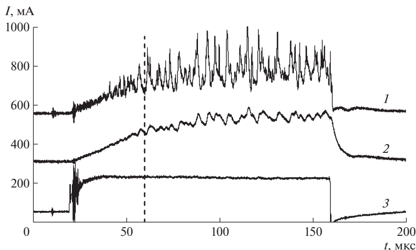
Рис. 3. Осциллограммы инвертированного зондового тока без ФНЧ — 1, с ФНЧ — 2, и тока разряда — 3. Штриховой линией показан момент измерения. Ток разряда 5 А, напряжение смещения 0 В, длина плазмы 20 см.
