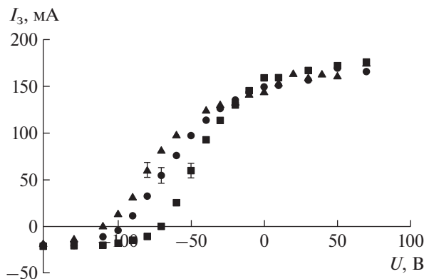
Рис. 7. Вольтамперные характеристики зонда для трех длин плазменного столба: 10 см (левая кривая), 20 см (средняя кривая) и 30 см (правая кривая). Горизонтальная погрешность меньше размера точки, вертикальная погрешность указана на графике для одной точки. Ток разряда 5 А.
