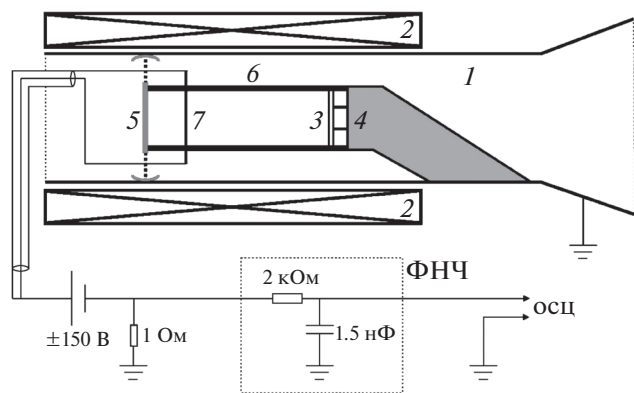
Рис. 1. Схема установки: 1 – волновод, 2 – соленоид, 3 – термокатод, 4 – электрод-держатель, 5 – подвижный коллектор, 6 – трубчатая плазма, 7 – зонд.
