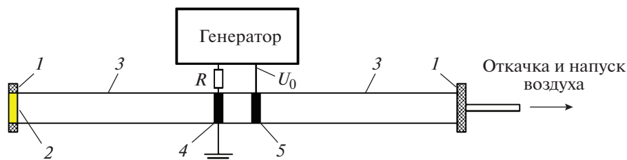
Рис. 1. Установка для изучения стримеров в ПДС, инициируемых емкостным разрядом. 1 – фланцы из капролона, 2 – кварцевое окно, 3 – трубка из кварца, 4 – заземленный кольцевой электрод на поверхности кварцевой трубки, 5 – высоковольтный электрод на поверхности кварцевой трубки. R – сопротивление шунта, U_0 – высоковольтный вывод генератора, к которому подключался делитель напряжения и электрод 5.
