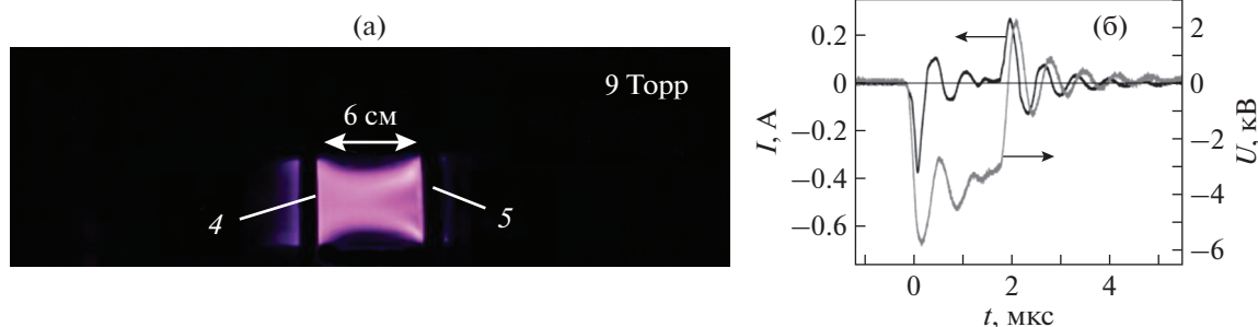
Рис. 2. Фотография разряда в трубке между электродами (а), а также осциллограммы импульсов напряжения U и тока разряда I (б). Давление воздуха p = 9 Торр. Напряжение генератора U_0 = -7 кВ.
