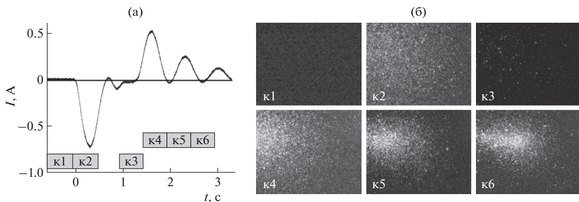
Рис. 8. Осциллограмма тока разряда, на временной шкале которой показаны места привязки отдельных кадров ICCD-камеры (к1, к2, к3) и (к4, к5, к6) во время двух импульсов с их длительностями (а), а также изображения свечения разряда шириной 3 см во время этих кадров, полученные на расстоянии 11 см от края правого (высоковольтного) электрода, который находился слева от изображений (б). Соответственно, все изображения были получены в области трубки между 11 и 14 см от края высоковольтного электрода. Длительность каждого из кадров равна 0.5 мкс. Излучение на кадре к2 наблюдается во время первого пика на импульсе тока, а на кадре к4 во время второго пика на импульсе тока. Задержка между пиками тока равнялась 1.3 мкс. U_0 = -6 кВ, p = 3.6 Торр.
