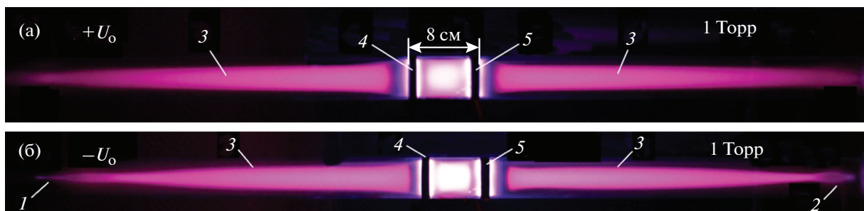
Рис. 4. Фотографии свечения ПДС в кварцевой трубке и емкостного разряда между электродами при U_0 = +7 (а) и -7 кВ (б). 1 и 2 — области формирования третьего стримера при отрицательной полярности импульса напряжения, 3 — ПДС, 4 — заземленный электрод, 5 — высоковольтный электрод. Давление воздуха p = 1 Торр. Экспозиции 0.2 с.
