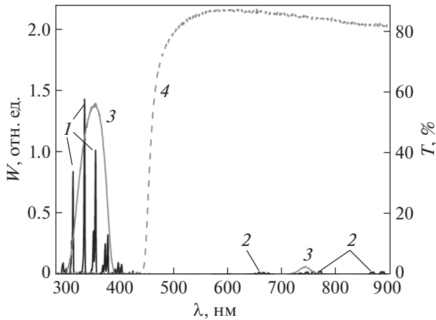
Рис. 7. Спектр излучения ПДС из области, расположенной на расстоянии 11 см от края правого электрода и области пропускания светофильтров. 1 – наиболее интенсивные полосы 2+ системы азота, 2 – наиболее интенсивные полосы 1+ системы азота, 3 – пропускание светофильтра УФС-5, 4 – пропускание светофильтра ЖС-16. p = 1 Торр, U_0 = +7 кВ, экспозиции 20 с.
