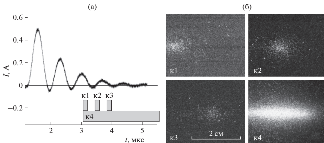
Рис. 10. Оциллограмма тока разряда, приведенная начиная со второго пика импульса тока, на временной шкале которой показаны места привязки отдельных кадров ICCD-камеры (к1, к2, к3, к4) и их длительности (а), а также изображения фронта третьего стримера на расстоянии от 53 до 56 см от правого электрода, который находился с левой стороны от изображений, полученных за 0.14 мкс (к1, к2 и к3) и 2.5 мкс (к4) (б). Ширина каждого изображения 3 см. Задержка между началом кадров к1 и к2, а также кадров к2 и к3 равнялась 0.4 мкс, кадры к1 и к4 начинались одновременно. Съемка была выполнена при одинаковой чувствительности для всех каналов ICCD-камеры. U_0 = -6 кВ, p = 1 Торр.
