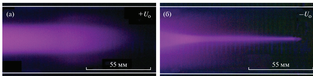
Рис. 5. Фотографии свечения ПДС у их окончания при напряжении генератора U_0 = +7 (а) и -7 кВ (б). Край правого электрода 5 (см. рис. 4) расположен слева от левого края фотографий этого рисунка на расстоянии 23 см. p = 1.5 Торр. Экспозиция 1 с.
