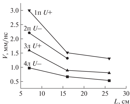
Рис. 9. Зависимости средней скорости фронта первых стримеров, распространяющихся от электродов вправо (1п, 2п) и влево (3л, 4л) при напряжении генератора +4.5 (1п, 3л) и -4.5 кВ (2п, 4л). Точки на зависимостях, которые расположены слева, соответствуют средней скорости прохождения фронтом области трубки от 3 до 11 см, средние точки – от 11 до 21 см и правые – от 21 до 31 см. Эти точки на кривых соответствуют серединам указанных выше областей, а L равняется расстоянию от края ближайшего электрода до середины данной области. p = 1 Торр.
