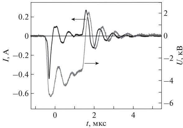
Рис. 3. Осциллограммы импульсов напряжения U и тока разряда I . Давление воздуха p = 1 Торр. Амплитуда импульса генератора U_0 = -7 кВ.
