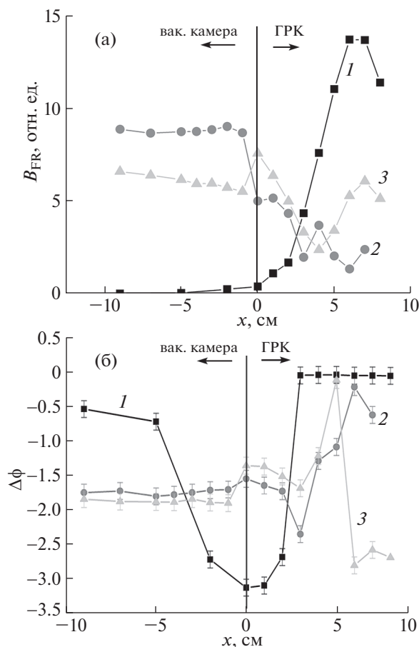
Рис. 15. Продольные распределения амплитуды B_{FR} (а) и сдвига фазы \Delta\phi (б) z -компоненты ВЧ магнитного поля для индуктивного разряда. Кривые 2, 3 построены для индукции постоянного магнитного поля 0 и 24 Гс соответственно. Кривая 1 описывает распределение без разряда (ВЧ-мощность 40 Вт).
