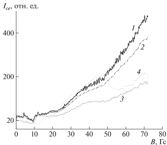
Рис. 11. Зависимость электронного тока I_{ee} на коллектор энергоанализатора без задерживающего напряжения от индукции магнитного поля. Номерами обозначены кривые для разных видов разряда: 1 – индуктивный, 2 – гибридный I, 3 – гибридный II, 4 – емкостной.
