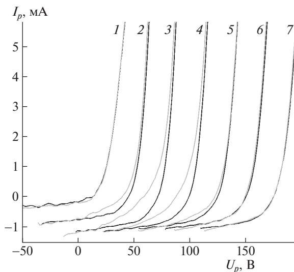
Рис. 12. Семейство ВАХ плоского зонда для его продольной (светлые кривые) и поперечной (темные кривые) ориентаций. Номера кривых соответствуют величинам индукции магнитного поля: 1 – 0 Гс, 2 – 15 Гс, 3 – 24 Гс, 4 – 36 Гс, 5 – 48 Гс, 6 – 60 Гс, 7 – 72 Гс.
