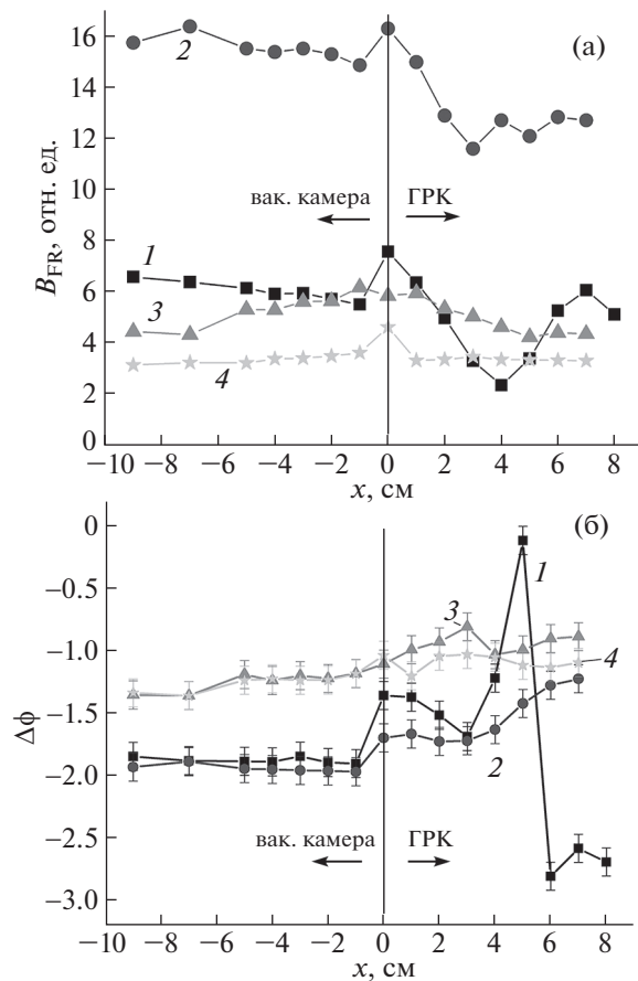
Рис. 16. Продольные распределения амплитуды B_{FR} (а) и сдвига фазы \Delta\phi (б) z -компоненты ВЧ магнитного поля. Номера обозначены кривые для разных видов разряда: 1 – индуктивный, 2 – гибридный I, 3 – гибридный II, 4 – емкостной.
