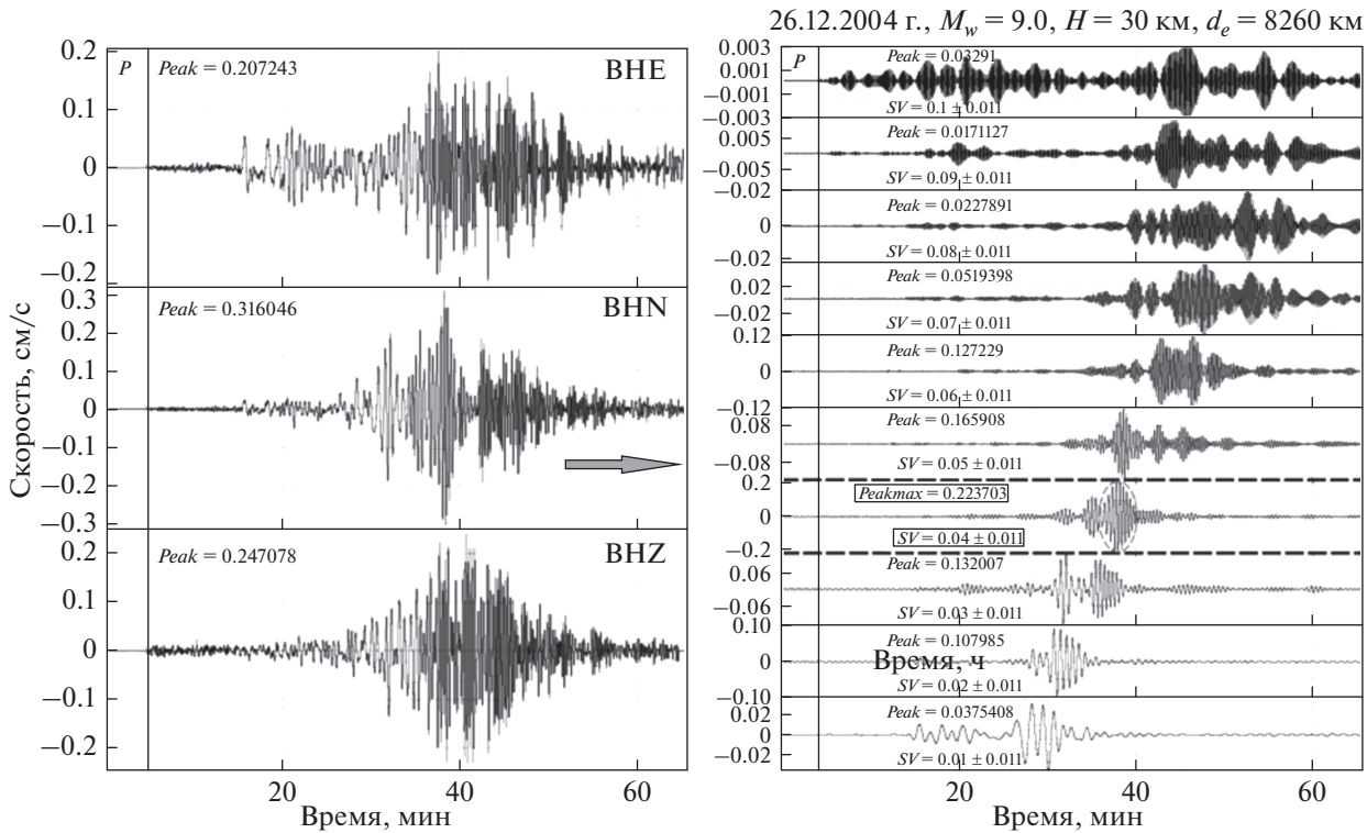
Рис. 8. Записи землетрясения 26.12.2004 г. (№ 3 в табл. 1, 2) на каналах BHE, BHN и BHZ, с/ст. PET с максимальными амплитудами Peak (левая диаграмма) и полосовая фильтрация записи скорости смещений грунта на канале BHN в программе DIMAS (правая диаграмма). Жирной пунктирной линией выделено ограничение частотной полосы SV = 0.04 \pm 0.011 Гц, в которой зафиксирована максимальная амплитуда скорости движений грунта Peakmax = 0.2237 см/с (выделена эллипсом).
