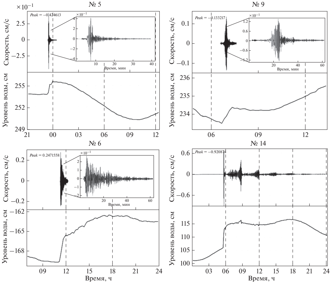
Рис. 4. Гидрогеосейсмические вариации уровня воды в скважине ЮЗ-5 (тип III), в сопоставлении с записями землетрясений на канале ВНЗ, с/ст. РЕТ. Номера землетрясений соответствуют табл. 1 и рис. 1.
