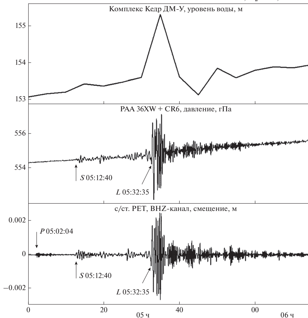
Рис. 6. Вариации уровня воды с периодичностью измерений 5 мин (Кедр ДМ) и давления подземных вод на глубине 5.6 м с частотой регистрации 10 Гц (датчик PAA 36XW) в скважине ЮЗ-5 при землетрясении 09.09.2017 г., M_w = 8.2 , Мексика (№ 19 в табл. 1) в сопоставлении с записью смещений на канале VHZ, с/ст. PЕТ.
