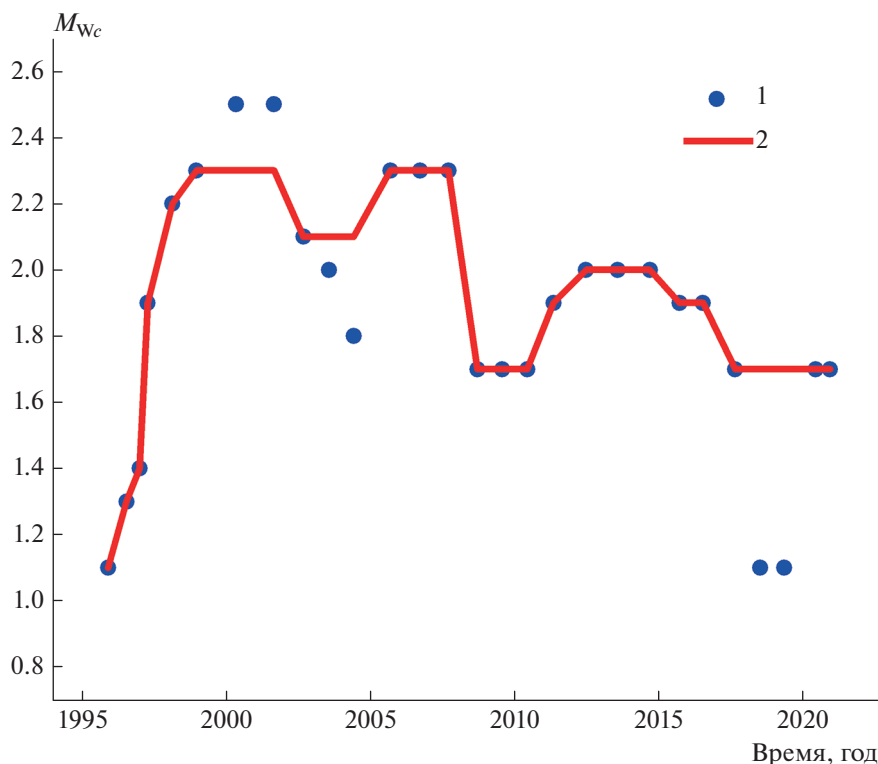
Рис. 2. Изменение представительной магнитуды во времени для каталога Исландии: 1 — исходные оценки, 2 — сглаженная кривая.
