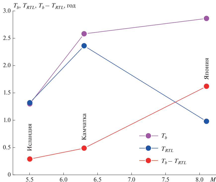
Рис. 7. Средние (медианые) длительности аномалий параметров b ( T_b ) и RTL ( T_{RTL} ) и их средняя (медианная) разность (по данным табл. 5).
