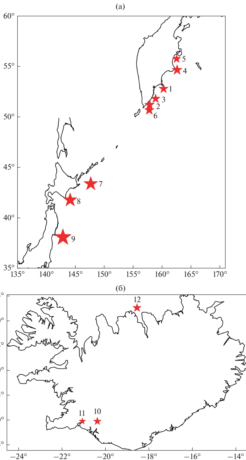
Рис. 3. Карты эпицентров отобранных землетрясений: (а) – Камчатка и Япония; (б) – Исландия. Размеры значков пропорциональны магнитуде, номера соответствуют табл. 1.
