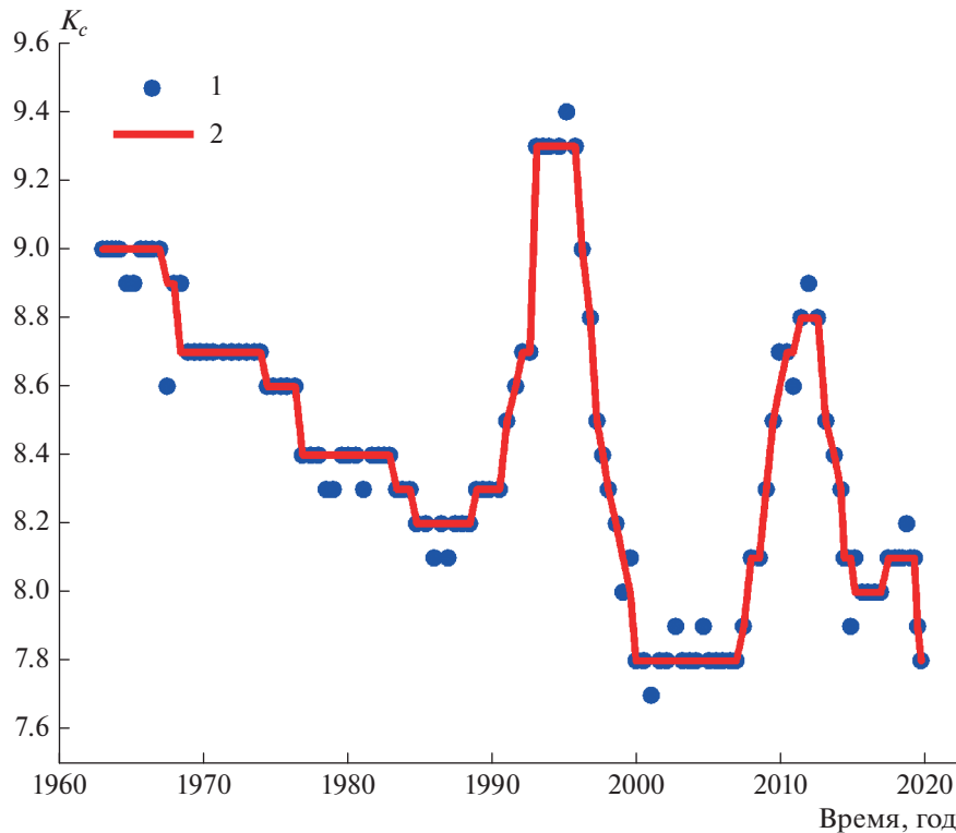
Рис. 1. Изменение представительного класса во времени для каталога Камчатки: 1 — исходные оценки, 2 — сглаженная кривая.
