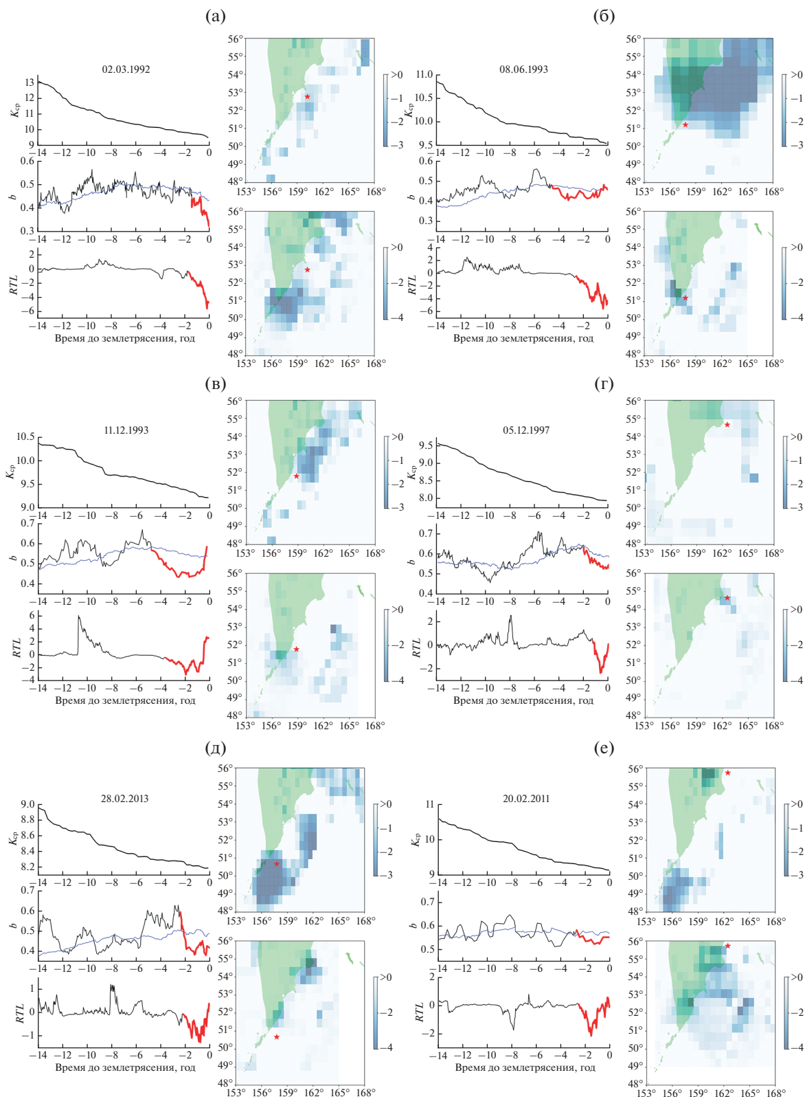
Рис. 4. Камчатка: карты распределения исследуемых параметров сейсмического режима в момент наибольшей величины аномалии и графики изменения значений параметров во времени. Карты: верхняя – параметр Z , нижняя – RTL ; звездочкой обозначен эпицентр землетрясений, масштаб цветовой шкалы показан справа от карт; (а)–(е) – различные землетрясения; над графиками подписаны их шифры в формате год_месяц_день, красным выделены аномалии. На графике параметра b тонкая линия – значения в фоновых окнах.
