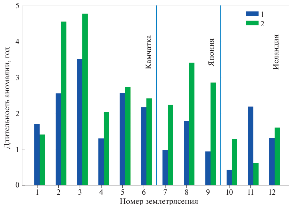
Рис. 6. Длительности аномалий: параметр RTL (1) и b (2), согласно табл. 4. По оси абсцисс – номер землетрясения согласно табл. 1.
