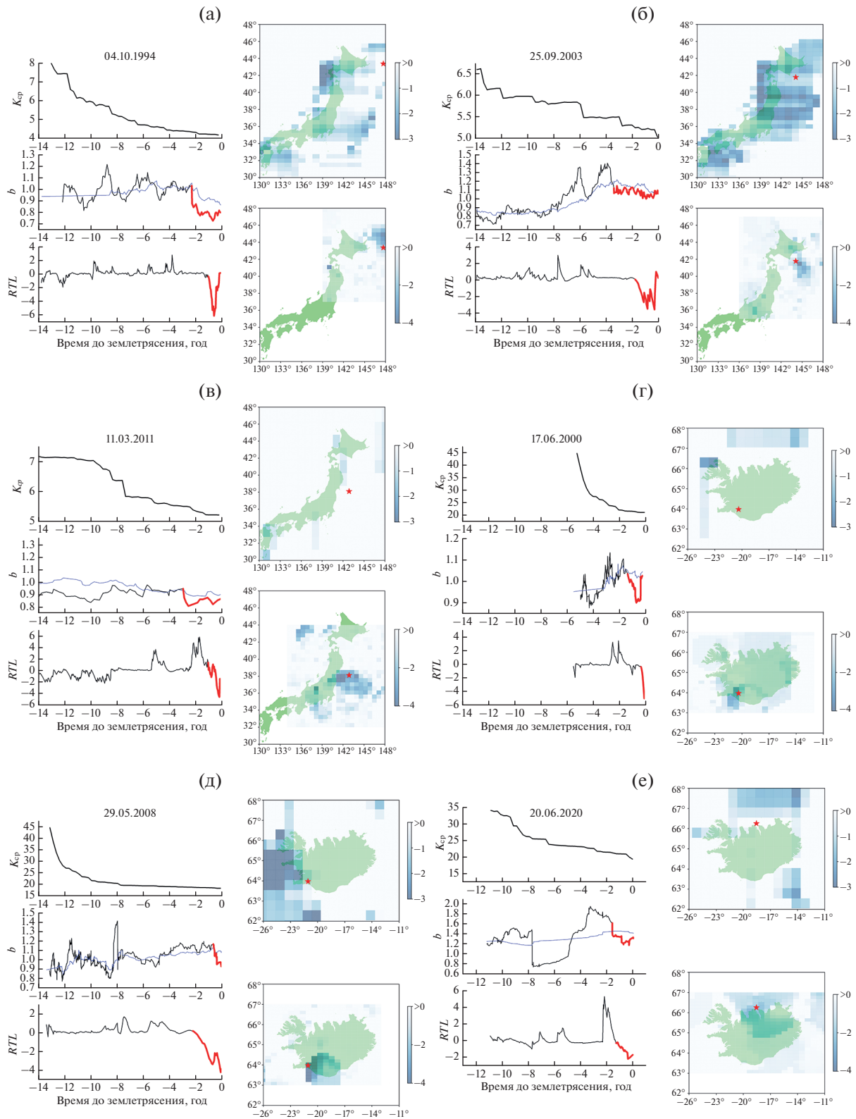
Рис. 5. Япония (а), (б), (в) и Исландия (г), (д), (е): карты распределения исследуемых параметров сейсмического режима в момент наибольшей величины аномалии и графики изменения значений параметров во времени. Обозначения – как на рис. 4.
