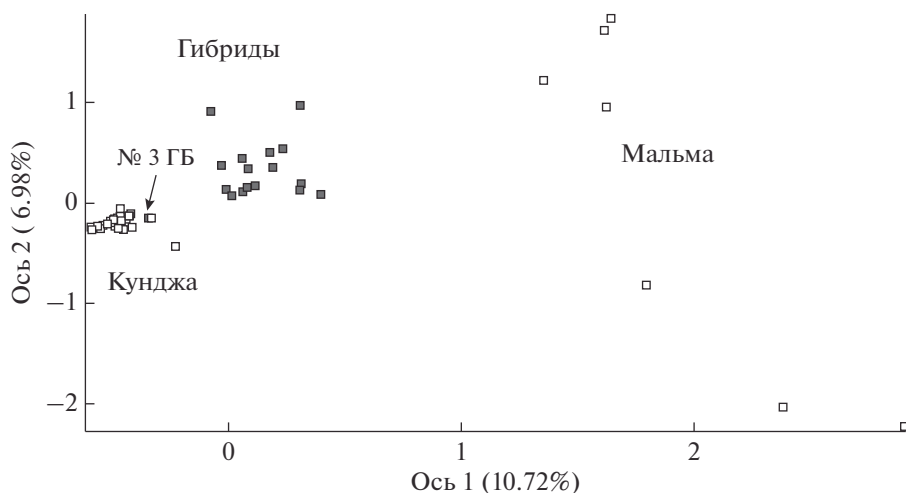
Рис. 1. Результаты факторного анализа в координатах двух осей для особей мальмы, кунджи и их гибридов из р. Утхолок, полученные на основе анализа генотипов по девяти микросателлитным локусам.
