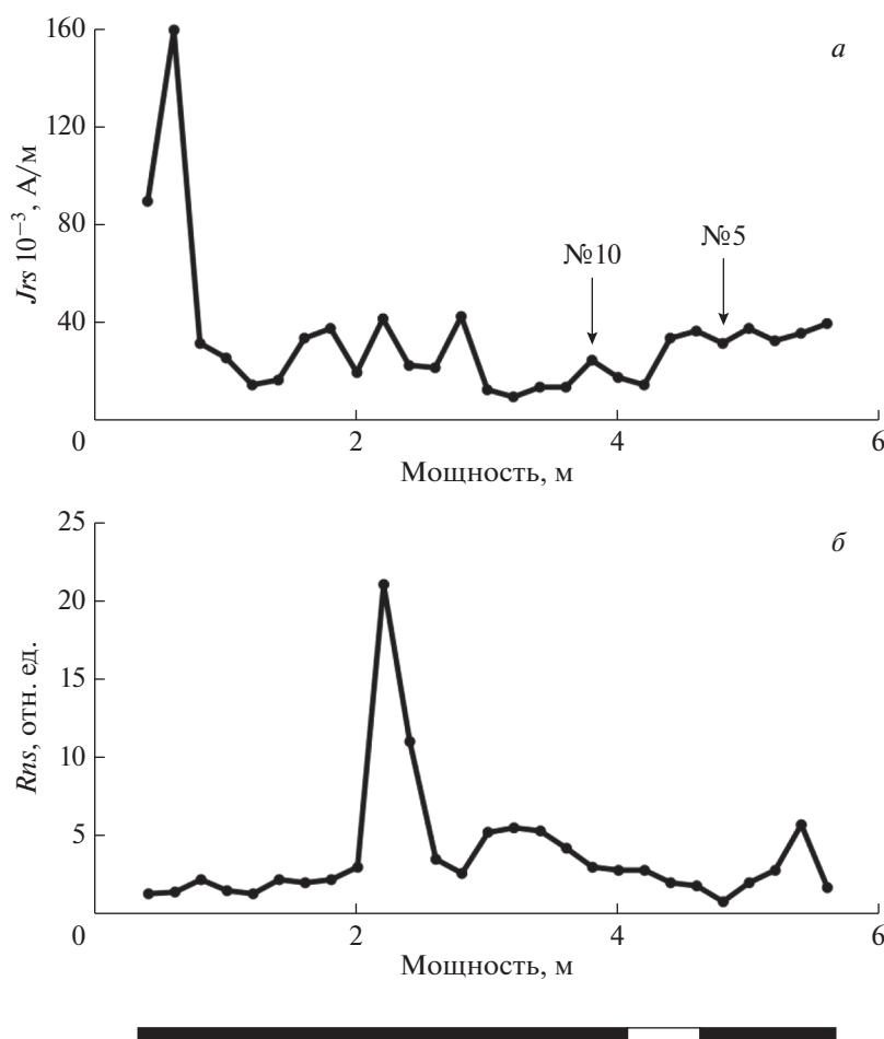
Рис. 3. Изменения Jrs по мощности отложений нижнего палеогена ( a ) и палеонапряженности Rms ( б ) по мощности осадочной толщи. Внизу черным цветом обозначена прямая полярность, белым цветом — обратная полярность геомагнитного поля.
