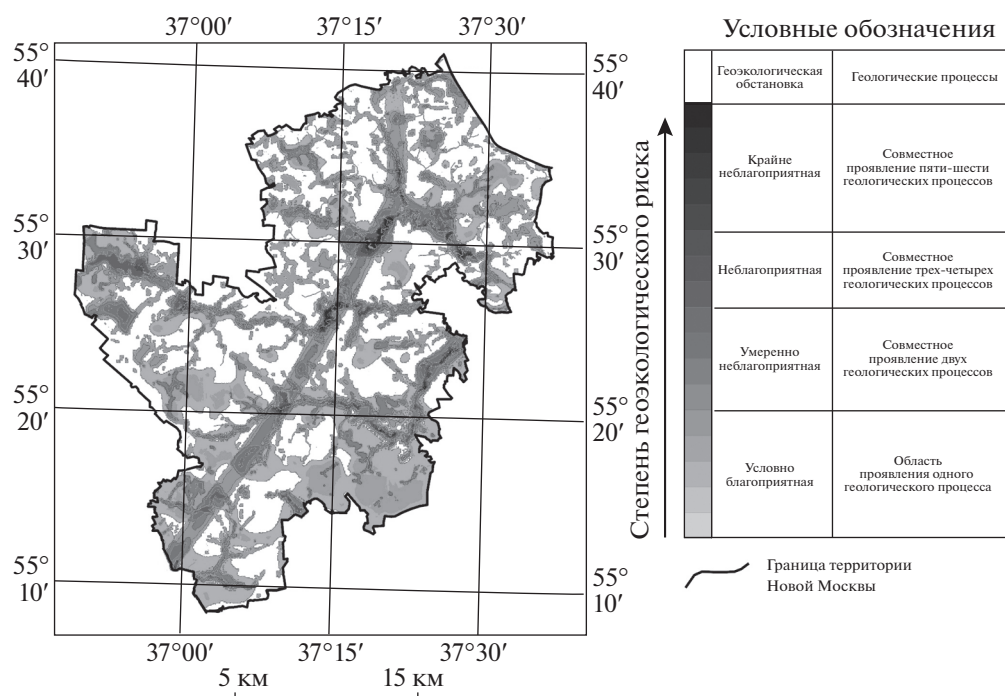
Рис. 1. Геоэкологическая карта территории Новой Москвы с учетом неблагоприятных геологических процессов и влияния неотектонического разлома.
