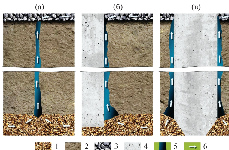
Рис. 2. Схемы, иллюстрирующие условия развития суффозионных процессов (фильтрационного разрушения и подземной эрозии) в основании строящегося здания при наличии: а – плохо затампонирующей разведочной скважины; б – неплотного примыкания грунта к “стене в грунте”, в местах ее погружения ниже подошвы водоупора; в – неплотного примыкания грунта к боковым поверхностям забитых свай. 1 – древесно-щебенистый грунт; 2 – суглинок (водоупор); 3 – материал пластового дренажа; 4 – бетон; 5 – сквозное нарушение сплошности водоупора, заполненное водой; 6 – направление потока подземных вод и транзита грунтовых частиц (в поровом пространстве пластового дренажа поток направлен в сторону водозаборного зумпфа).
