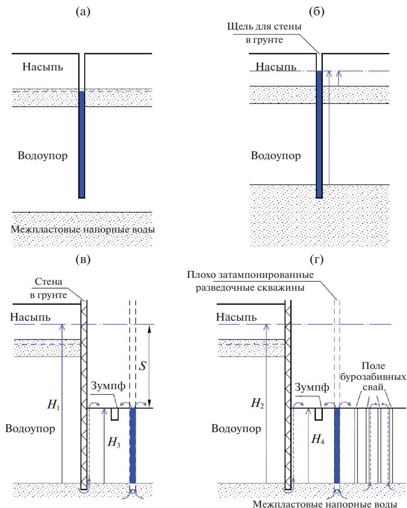
Рис. 3. Схематическое отражение изменения гидрогеологических условий на участке в процессе строительства подземной части объекта: а – не достиг подошвы водоупора; б – вскрывает кровлю напорного водоносного горизонта; в – в период разработки котлована; г – после сооружения свайного поля под высотными корпусами здания. H_1 и H_2 – высота напора подземных вод, за пределами “стены в грунте” при работающем насосе в зумпфе; H_3 и H_4 – высота напора подземных вод на момент включения и выключения насоса в зумпфе; S – величина водопонижения.
