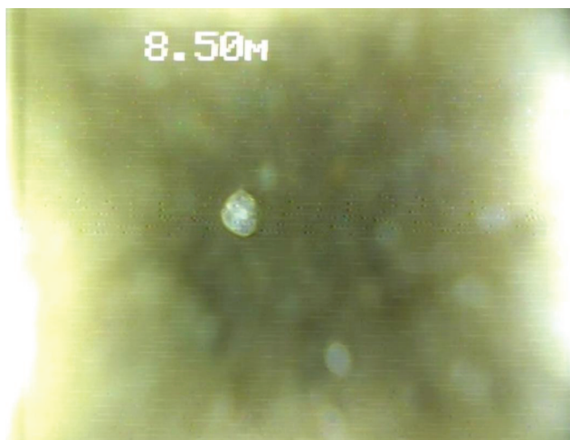
Рис. 6. Плавающая гравийная частица в открытой скважине на высоте 1.3 м выше кровли напорного водоносного горизонта.
