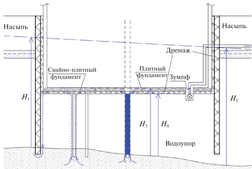
Рис. 4. Существующие гидрогеологические условия на участке строительства после сооружения пластового дренажа, фундаментной плиты и зумпфа, откачивающего воду из дренажной системы. H_1 и H_2 — высота напора подземных вод, за пределами «стены в грунте» при работающем насосе в зумпфе; H_3 и H_4 — высота напора подземных вод на момент включения и выключения насоса в зумпфе.
