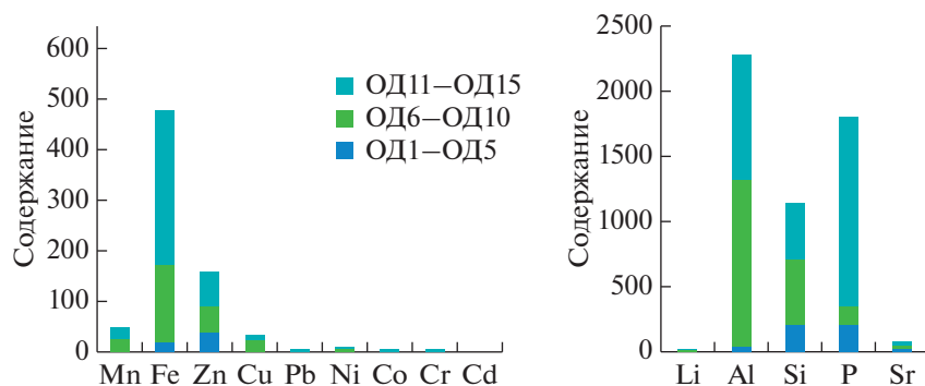
Рис. 5. Гистограмма с накоплением средних содержаний халькофильных и литофильных химических элементов в конденсационных водах над отходами добычи руд (мкг/л). Условные обозначения: ОД1–ОД5, ОД6–ОД10, ОД11–ОД15 – наименования профилей.
