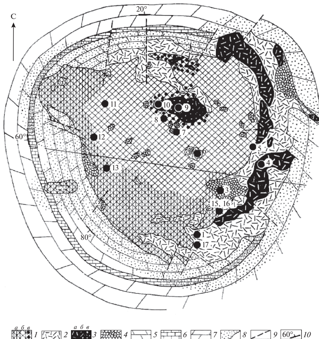
Рис. 2. Схематическая геологическая карта интрузии Одихинча (Егоров, 1969) с точками отбора пород. Номера образцов указаны без индекса Od (табл. 1). Условные обозначения: 1 – ийолиты-мельтейгиты (а – мельтейгиты, б – ийолиты, ийолит-уртиты, в – меланитовые ийолиты), 2 – якупирангиты-мельтейгиты, 3 – мелилитовые породы (а – ункопагриты, б – турьяиты, в – окаиты), 4 – оливиниты, 5 – доломиты среднего кембрия, 6 – известняки нижнего кембрия, 7 – доломиты верхнего кембрия, 8 – ореол контактового метаморфизма, 9 – разломы, 10 – залегание осадочных пород.
