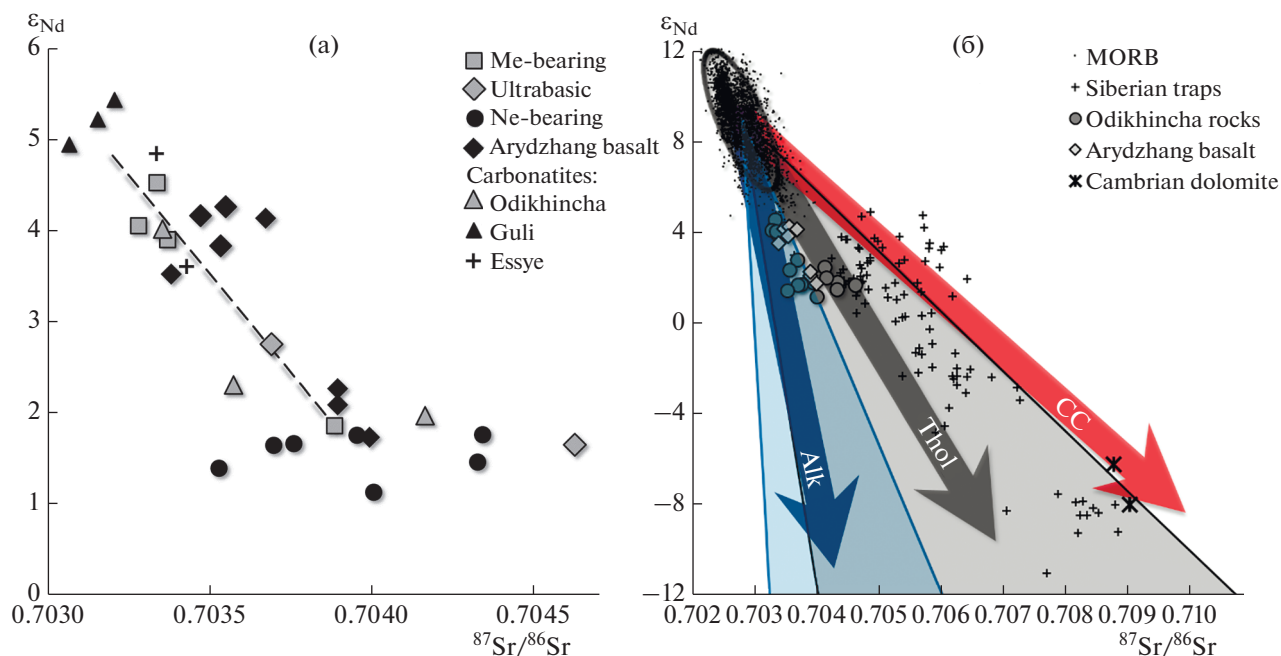
Рис. 5. Изотопные отношения неодаима (в виде \epsilon_{Nd}(T) ) и стронция (а) — в мелилит-содержащих (Me-bearing), нефелин-содержащих (Ne-bearing), ультраосновных породах и карбонатитах массива Одихинча, а также карбонатитах массивов Ессей (Essey) и Гули (Guli) (Morikyo et al., 2001), и щелочных базальтах арыджангской свиты, включая данные (Fedorenko et al., 2000). Пунктирная линия отвечает кривым на рис. 7; (б) — те же данные в сравнении с данными (Костицын, 2004, 2007) по базальтам срединно-океанических хребтов (MORB) и Сибирским траппам (Lightfoot et al., 1993; Wooden et al., 1993; Hawkesworth et al., 1995; Arndt et al., 1998; Krivolutsкая et al., 2012; Kiselev et al., 2014; Reichow et al., 2016), также использованы неопубликованные данные Ю.А. Костицына и Н.А. Криволуцкой. Показаны составы вмещающих массив среднекембрийских доломитов (табл. 5). Для MORB приведен двухсигмовый эллипс их разброса. Широкими стрелками указано возможное положение древних обогащенных источников изначально мантийного изотопного состава, но с элементными характеристиками (Rb/Sr и Sm/Nd), отвечающими континентальной земной коре (Taylor, McLennan, 1985) — CC (красная стрелка), медианным составом толеитовых базальтов и габбро — Thol (серая стрелка) и щелочных пород — Alk (синяя стрелка). Для последних двух групп пород показаны поля с учетом гетерогенности Rb/Sr и Sm/Nd отношений в них (табл. 5) так же серым и синим цветами).
