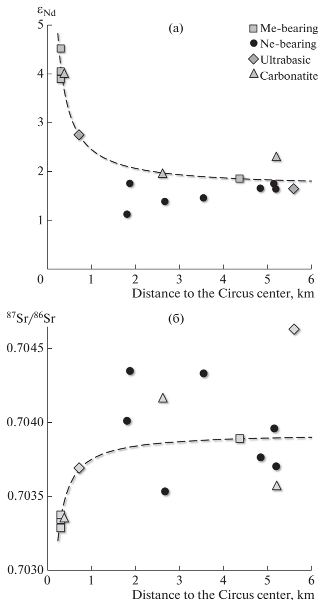
Рис. 7. Зависимость начальных изотопных отношений неодиима (а) и стронция (б) от расстояния до центральной части цирка на горе Одихинча. Мелилит-содержащие (Me-bearing) породы на обоих графиках образуют гиперболическую кривую, к которой отчасти тяготеют карбонатиты и ультраосновные породы, тогда как нефелин-содержащие (Ne-bearing) породы не следуют этой географической зависимости.
