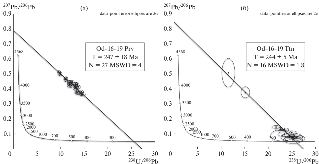
Рис. 4. Диаграммы Тера-Вассербурга с результатами анализа кристаллов перовскита (а) и титанита (б) из карбонатита Od-16-19 массива Одихинча.
