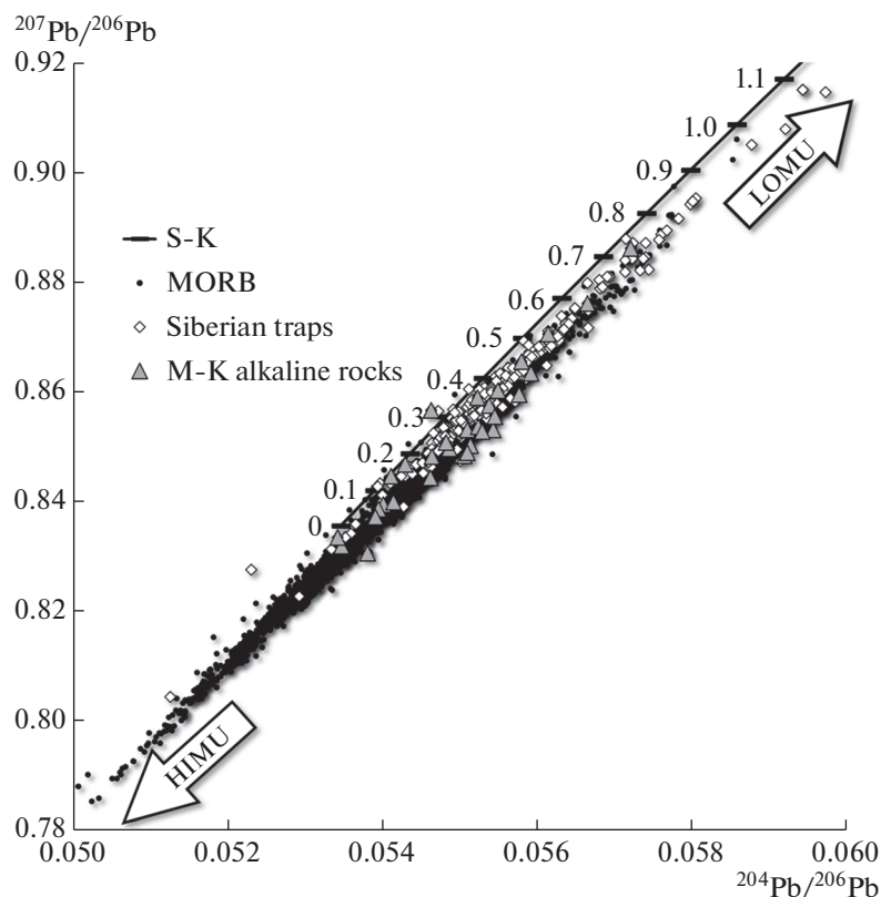
Рис. 6. Вариации изотопного состава свинца в Сибирских траппах (Sharma et al., 1992; Lightfoot et al., 1993; Wooden et al., 1993; Czamanske, 2002; Arndt et al., 2003; Carlson et al., 2006; Krivolutsкая, Rudakova, 2009; Малич и др., 2010; Krivolutsкая et al., 2012) и щелочных породах маймеча-котуйского комплекса ( M-K alkaline rocks ) (Sharma et al., 1992; Carlson et al., 2006; Kogarko, Zartman, 2007). Для сравнения приведены также данные для базальтов срединно-океанических хребтов (MORB) из работ (Костицын, 2004, 2007) и состав модельного источника (S-K) по (Stacey, Kramers, 1975). Цифры около кривой отвечают модельному возрасту свинца в млрд лет по модели Стейси-Крамерса. Показаны также направления на составы источников с высокими (HIMU) и низкими (LOMU) отношениями U/Pb.
