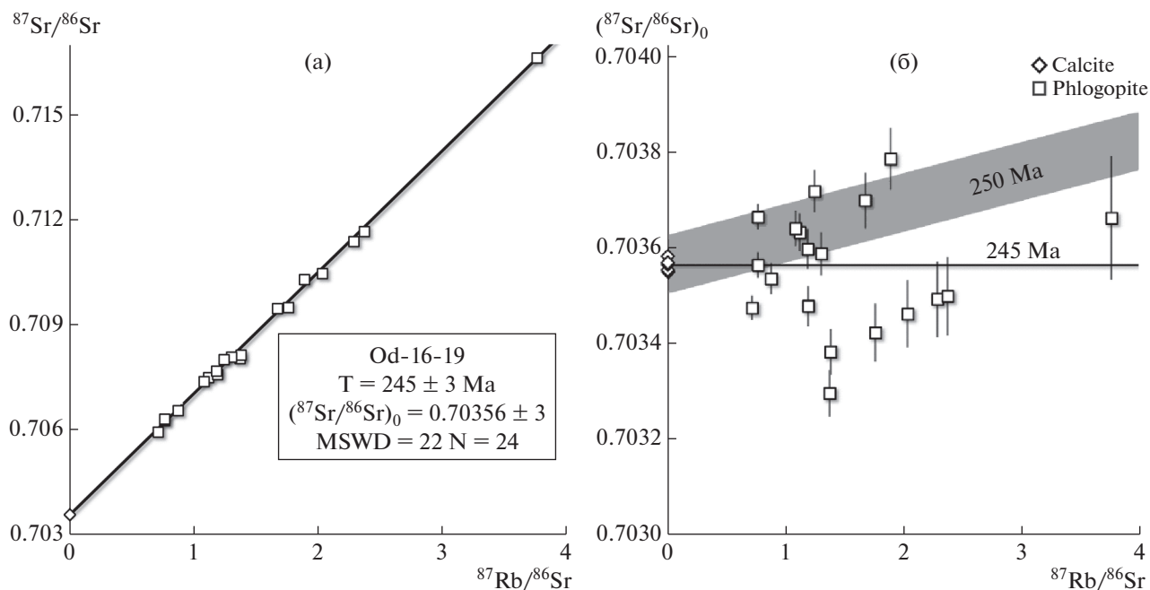
Рис. 3. Изохронная диаграмма (а) для карбонатита Od-16-19 по отдельным зернам кальцита и флогопита, и “график остатков” (б) для этих же данных. Rb–Sr система минералов нарушена и расположение аналитических точек не противоречит тому, что возраст карбонатита близок к 250 млн лет.
