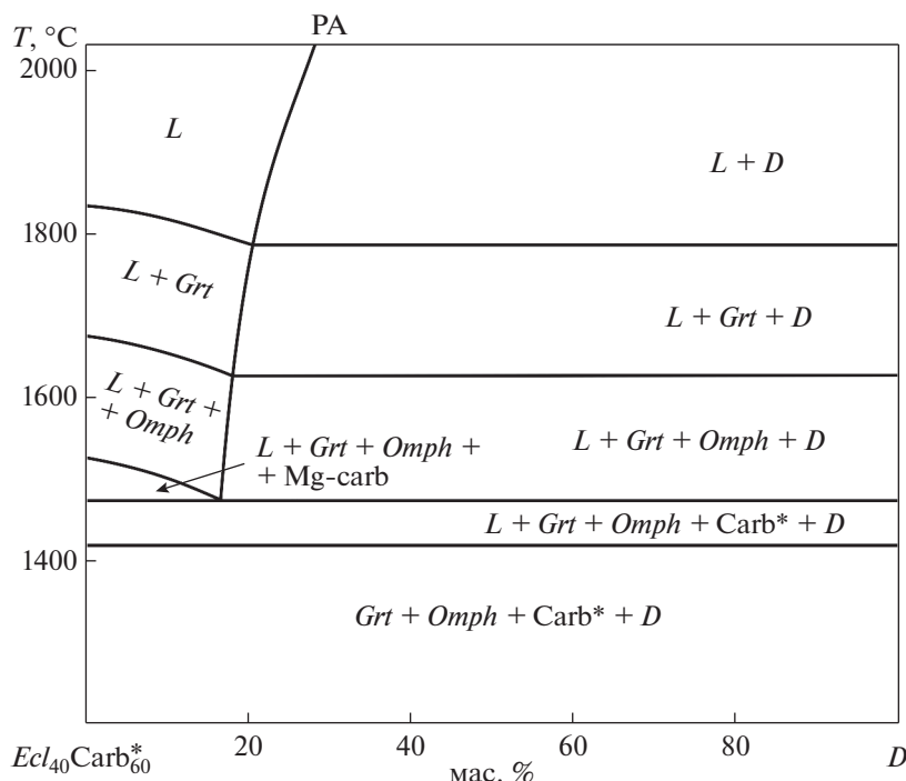
Рис. 5. Равновесная диаграмма сингенезиса алмаза и ассоциированных фаз базитовой системы эклогит–карбонат Carb*–углерод С (= алмаз D) в ее политермическом сечении Ecl 40 Carb* 60 – D по данным эксперимента при 7.0 ГПа. Символы: PA – кривая растворимости алмаза, L – полностью смешимый карбонат-силикатный расплав, Ecl – эклогит, Mg-carb – Mg-карбонат, Carb* – объединенный символ карбонатов Mg, Fe, Ca, Na для упрощения диаграммы, Omph – омфациит, Grt – гранат, D – алмаз.
