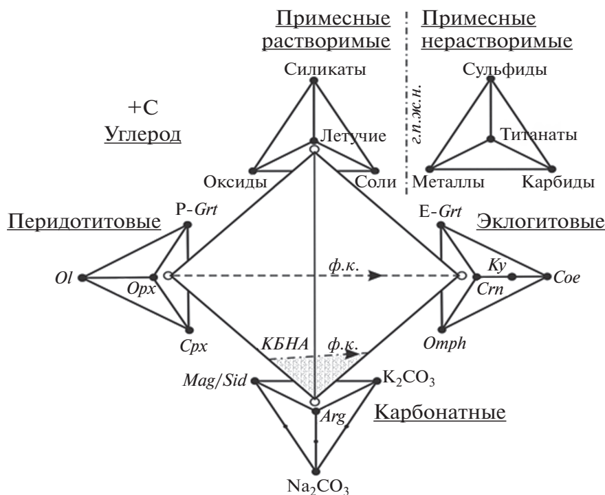
Рис. 7. Обобщенная диаграмма-тетраэдр составов материнских расплавов алмазов и ассоциированных фаз (заштрихованная область). Условные обозначения: Ol – оливин, Opх – ортопироксен, Срх – клинопироксен, P-Grt гранат перидотитового парагенезиса, Omph – омфакит, E-Grt – гранат эклогитового парагенезиса, Crn – корунд, Ku – кианит, Coe – коэсит, Mag – магнезит, Arg – арагонит, Sid – сидерит, – КБНА – концентрационный барьер нуклеации алмаза, г.п.ж.н. – граница полной жидкостной несмесимости, ф.к. – фракционная кристаллизация, направление которой обозначено стрелкой.
