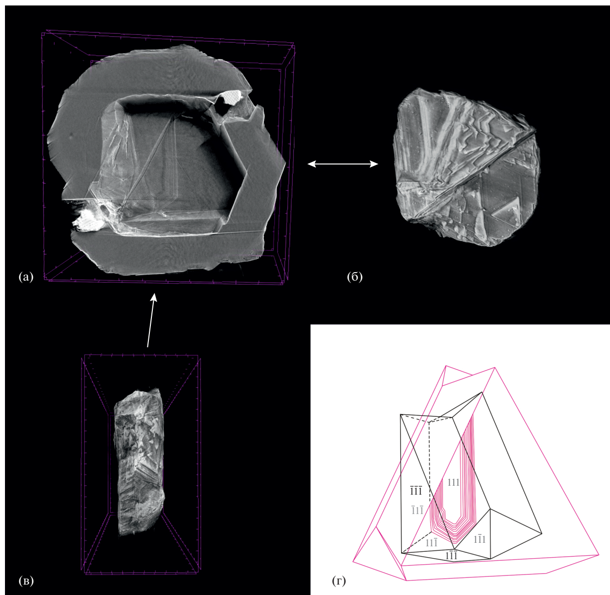
Рис. 2. Схема совмещения томографических изображений футляра и ядра алмаза “Матрешка” по следам совместного роста в виде штриховки граней индукции: (а) продольное сечение футляра алмаза и стенка полости со следами индукции (Коногорова и др., 2020); (б) ядро алмаза со следами индукции; (в) ориентировка алмазного ядра относительно стенки футляра; (г) схема совмещения контактных двойников, слагающих футляр и ядро алмаза с проекцией секторов роста граней октаэдра и розетки, с индукционной штриховкой (символы лицевых граней показаны черным цветом, а с противоположной стороны – серым).
