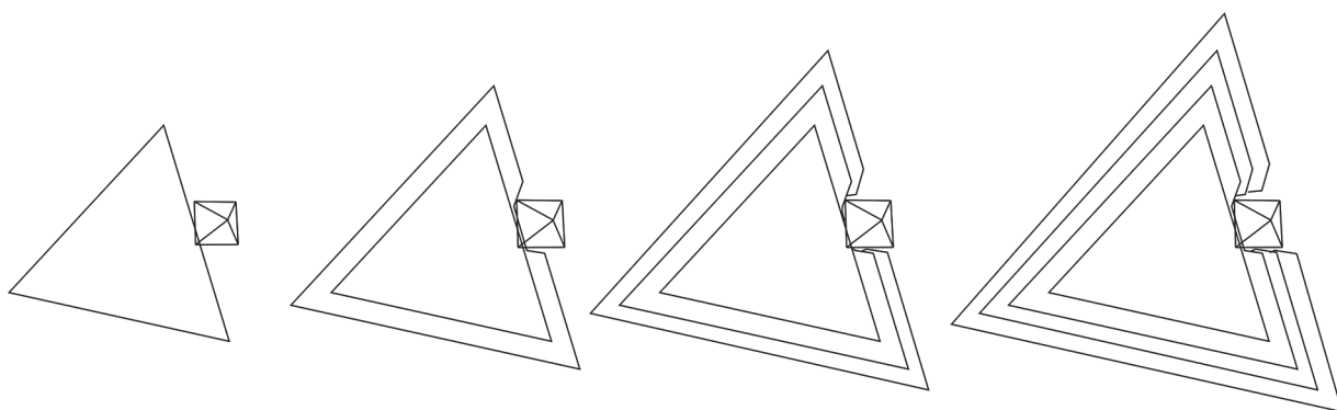
Рис. 8. Схема захвата индивида алмаза двойниковой границей двугранного внешнего угла во время роста шпинелевого двойника, и образование полости вокруг кристалла.
