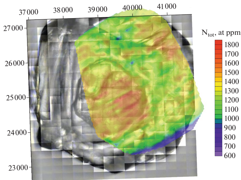
Рис. 4. Распределение суммарной концентрации азота ( N_{tot} ) в алмазе “Матрешка”.
