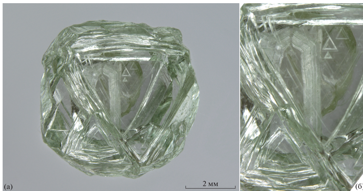
Рис. 1. Индукционная штриховка на внутренней стенке полости футляра алмаза “Матрешка”, проходящий свет.
