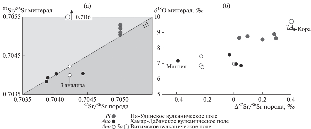
Рис. 9. Диаграмма соотношений (а) ^{87}\text{Sr}/^{86}\text{Sr} в минералах и несущих их породах и (б) отклонения изотопных соотношений ^{87}\text{Sr}/^{86}\text{Sr} от линии 1 : 1 ( \Delta^{87}\text{Sr}/^{86}\text{Sr} ) напротив измеренных \delta^{18}\text{O} в полевых шпатах.
