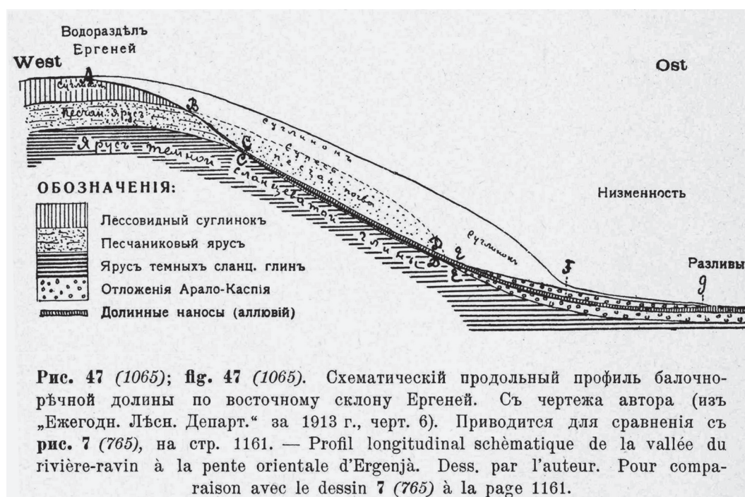
Рис. 1. Схематический продольный профиль балочно-речной долины восточного склона Ергеней. Обозначения на рисунке составил Г.Н. Высоцкий [10, рис. 47, стр. не указана, приложение].
