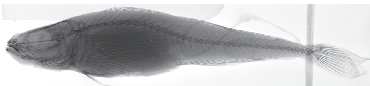
Рис. 3. Осевой скелет Cottocomephorus grewingkii BMNH 1897.7.5.4, синтип.
