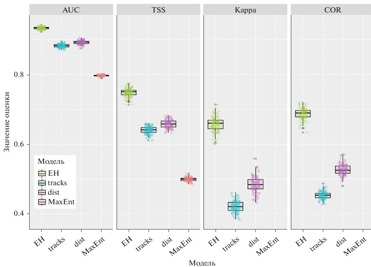
Рис. 3. Оценки качества моделей пространственного распределения черники на территории Центрально-Лесного заповедника и его охранный зоны для дизайнов GLM на основе подхода Энглера-Хенгла (EH), пройденных маршрутов (tracks), расстояний до точек присутствия (dist), а также для максимальной энтропии (MaxEnt).
