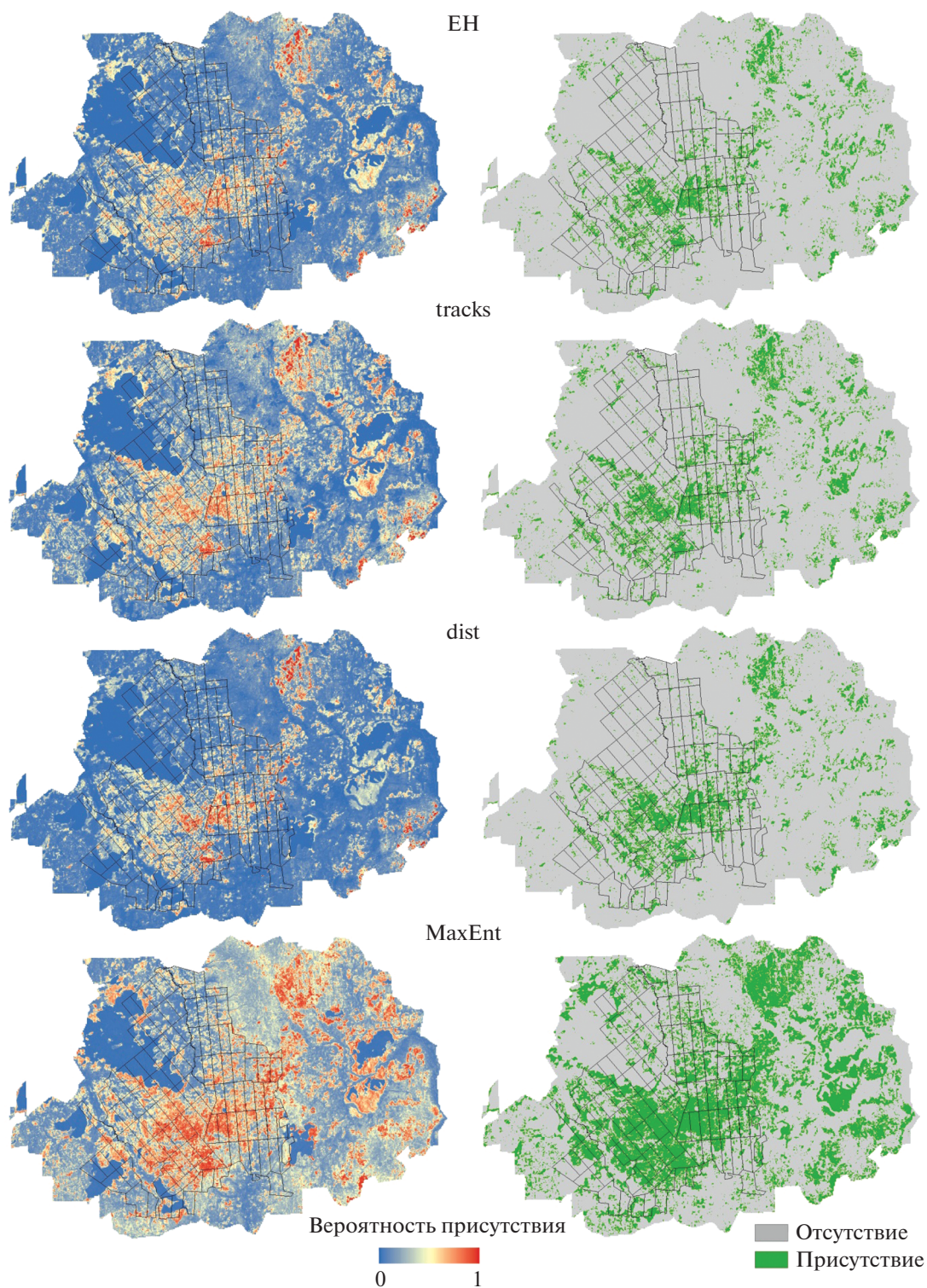
Рис. 5. Карты пространственного распределения черники на территории Центрально-Лесного заповедника и его охранный зоны для дизайнов GLM на основе подхода Энглера-Хенгла (ЕН), пройденных маршрутов (tracks), расстояний до точек присутствия (dist), а также для максимальной энтропии (MaxEnt). Слева карты непрерывных вероятностей присутствия, справа — классифицированные по выбранному порогу.
