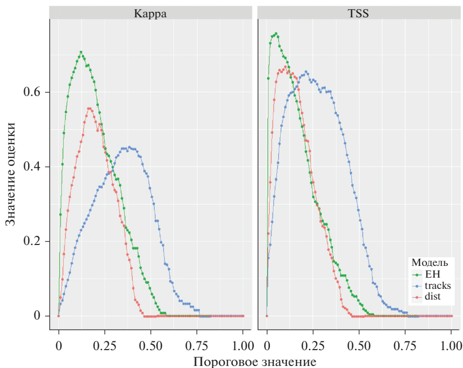
Рис. 4. Вариация значений Кappa и TSS в зависимости от пороговых значений для моделей пространственного распределения черники на территории Центрально-Лесного заповедника и его охранный зоны для дизайнов GLM на основе подхода Энглера-Хенгла (ЕН), пройденных маршрутов (tracks), расстояний до точек присутствия (dist).
