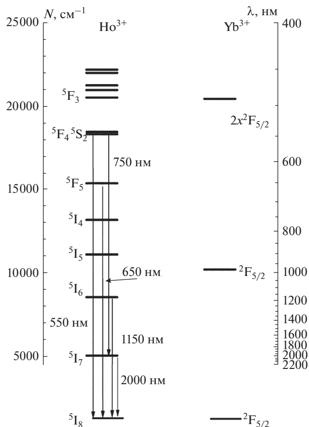
Рис. 1. Схема уровней ионов \text{Ho}^{3+} и \text{Yb}^{3+} и наблюдаемых переходов в кристаллах \text{MeF}_2-\text{Yb}-\text{Ho} . Показано также положение удвоенного по энергии уровня {}^2\text{F}_{5/2} \text{Yb}^{3+} .
