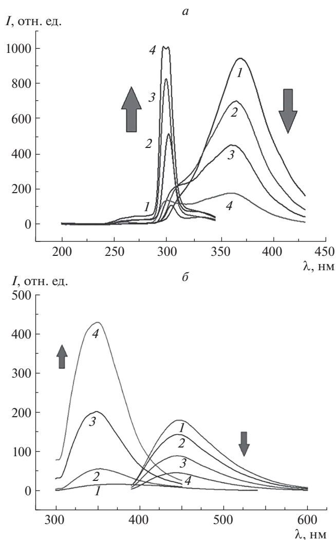
Рис. 1. a – Спектры возбуждения раствора альбумина при концентрации C = 0.1 \text{ мг} \cdot \text{мл}^{-1} (1), 0.05 \text{ мг} \cdot \text{мл}^{-1} (2), 0.025 \text{ мг} \cdot \text{мл}^{-1} (3), 0.0125 \text{ мг} \cdot \text{мл}^{-1} (4). б – спектры люминесценции раствора альбумина при концентрации C = 0.1 \text{ мг} \cdot \text{мл}^{-1} (1), 0.05 \text{ мг} \cdot \text{мл}^{-1} (2), 0.025 \text{ мг} \cdot \text{мл}^{-1} (3), 0.0125 \text{ мг} \cdot \text{мл}^{-1} (4).
