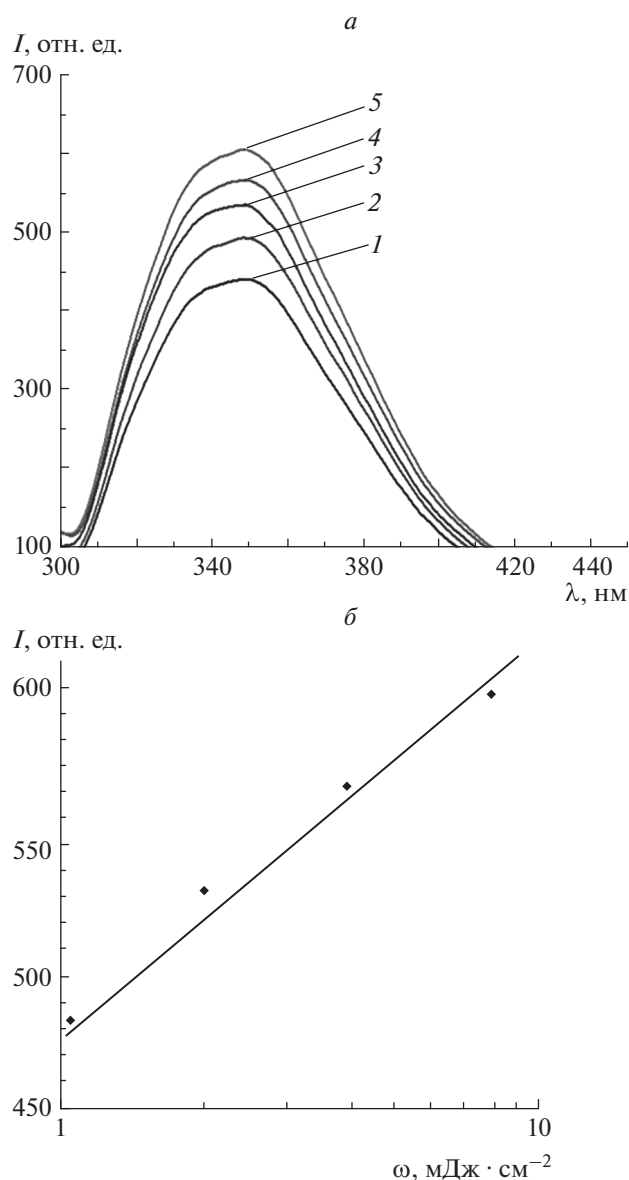
Рис. 4. a – Спектры люминесценции водного раствора альбумина при концентрации 0.0125 \text{ мг} \cdot \text{мл}^{-1} ; плотность мощности: 1 – без облучения, 2 – 1 \text{ мВт} \cdot \text{см}^{-2} , 3 – 2 \text{ мВт} \cdot \text{см}^{-2} , 4 – 4 \text{ мВт} \cdot \text{см}^{-2} , 5 – 8 \text{ мВт} \cdot \text{см}^{-2} . б – зависимость интенсивности люминесценции альбумина от плотности мощности облучения при постоянной плотности энергии.
