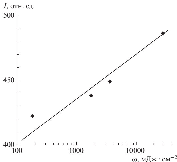
Рис. 3. Зависимость интенсивности люминесценции альбумина от плотности энергии облучения при постоянной плотности мощности.
