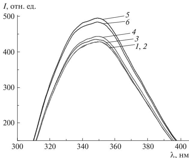
Рис. 2. Спектры люминесценции водного раствора альбумина при концентрации 0.0125 \text{ мг} \cdot \text{мл}^{-1} . Время облучения: 1 – 0, 2 – 180, 3 – 1800, 4 – 3600, 5 – 28800, 6 – 39600 с.
