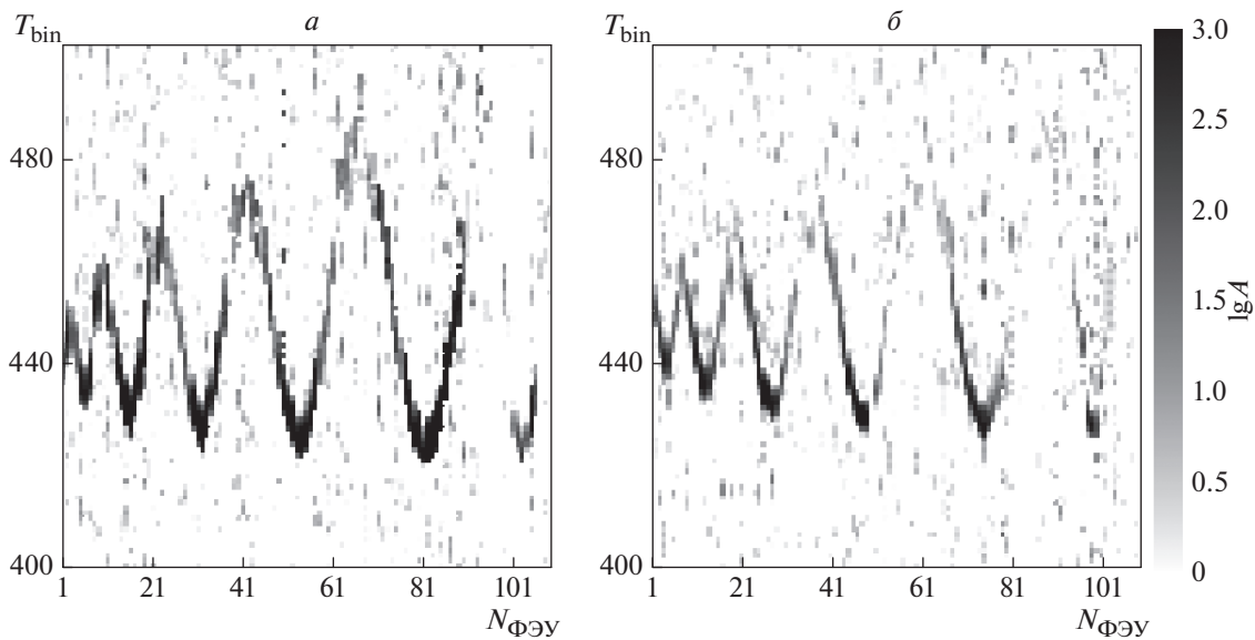
Рис. 1. Примеры отклика детектора СФЕРА-2: a – рассчитанный отклик установки, находящейся на высоте 580 м над уровнем наблюдения на черенковский свет от ядра железа с энергией 30 ПэВ; б – событие, зарегистрированное установкой в эксперименте 2013 г. с высоты 589 м.
