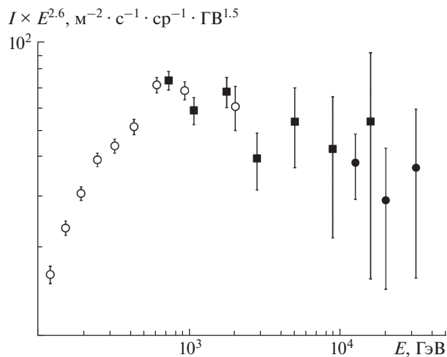
Рис. 2. Спектр никеля (энергия на частицу) поданным экспериментом НУКЛОН (квадратики – данные калориметра, кружки – данные KLEM) и по результатам HEAO-3-C2 [9].
