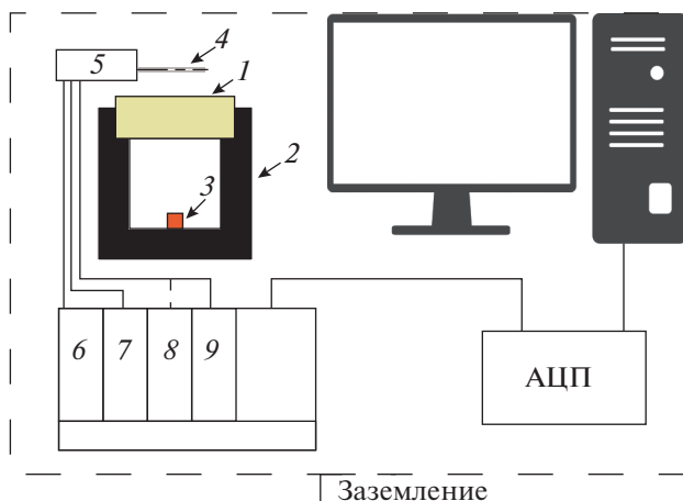
Рис. 2. Экспериментальная установка. 1 – термоллизатор, 2 – контейнер, 3 – источник, 4 – счетчик СНМ-50, 5 – предусилитель, 6 – низковольтное питание, 7 – высоковольтное питание, 8 – цифровой счетчик, 9 – спектрометрический усилитель.
