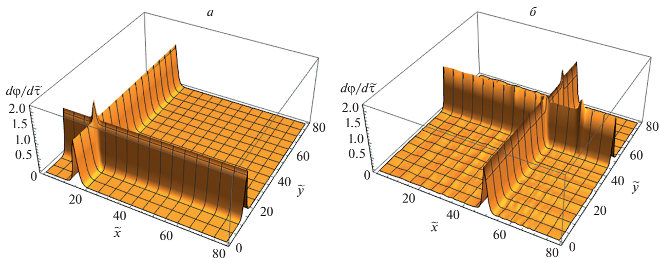
Рис. 1. Взаимодействие солитонов для \tilde{t} = 0 (а), 60 (б).
