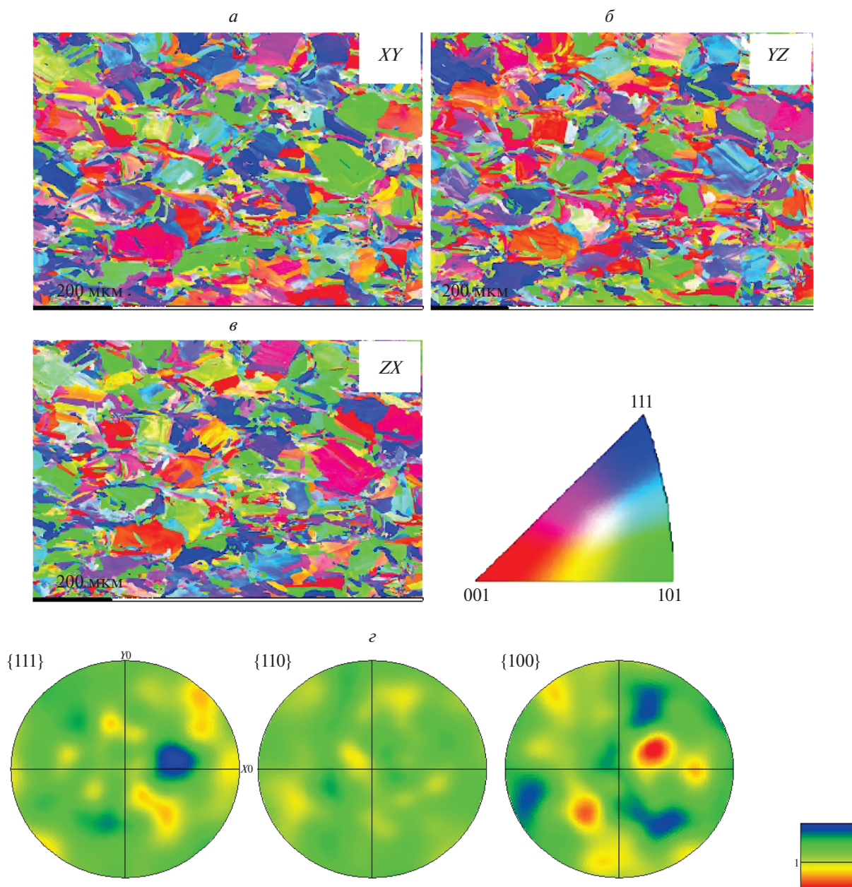
Рис. 3. Результаты текстурного анализа ЛС образца, EBSD-анализ, сканирующая электронная микроскопия: различные ориентации образца ( a–в ), ось z – направление роста образца в камере 3D принтера; полюсные фигуры ( з ).
