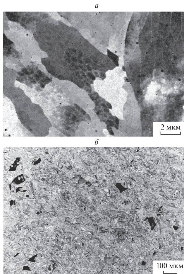
Рис. 1. Микроструктура ЛС образца, сканирующая электронная микроскопия: ячеисто-дендритная структура (а); участок образца с порами (б).
