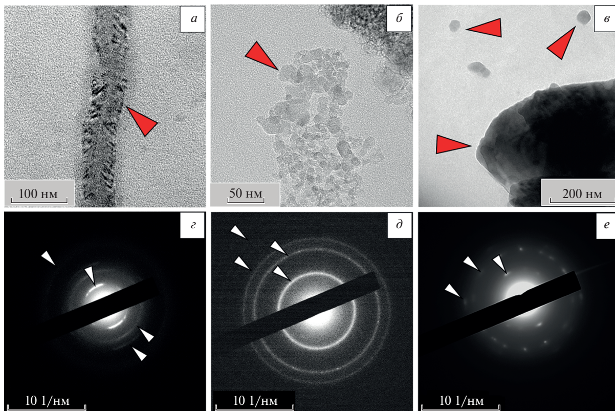
Рис. 1. Сравнение электронограмм разных типов УНЧ. Одиночная МУНТ (а), скопление наночастиц алмаза (б), кластеры наночастиц фуллерена C_{60} (в). Наночастицы показаны красными стрелками. ТЭМ. Электронограммы, полученные для а, б, в, соответственно (з, д, е). Белыми стрелками показаны дифракционные кольца. Дифракция электронов.
