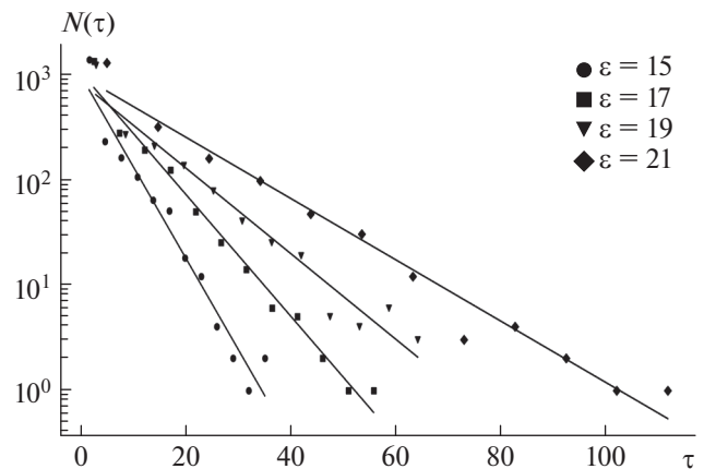
Рис. 1. Распределения длительностей ламинарных фаз N(\tau) двух однонаправленно связанных систем Лоренца (5), полученные при различных значениях параметра связи \varepsilon , и соответствующие им аппроксимации экспоненциальным законом (3): \varepsilon = 15 (●), \varepsilon = 17 (■), \varepsilon = 19 (▼), \varepsilon = 21 (◆).
