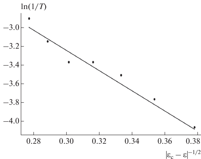
Рис. 2. Зависимость средней длительности ламинарных \ln(1/T) фаз от параметра надкритичности |\epsilon_c - \epsilon|^{-1/2} , полученная для двух однонаправленно связанных систем Лоренца (5), и ее аппроксимация закономерностью (4).
