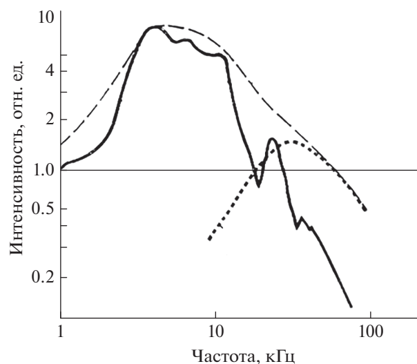
Рис. 1. Спектр радиоволн, излучаемых разрядом молнии. Сплошная линия – спектр основного разряда, точечный пунктир – спектр предразряда, штриховой пунктир – суммарный спектр.
