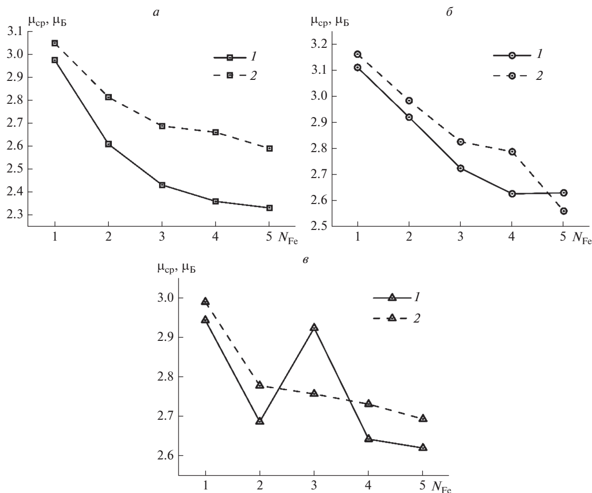
Рис. 2. Значение усредненного магнитного момента в зависимости от толщины пленки железа, для граней (100) ( a ), (110) ( б ), (111) ( в ); без релаксации (1), с релаксацией (2).
