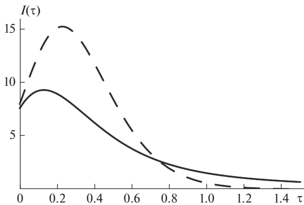
Рис. 1. Безразмерная интенсивность сверхизлучения в винеровском (пунктир) и невинеровском (сплошная линия) случаях. Положено \eta_+ = -\eta_- = \pi/4 , N_p = 8 .
