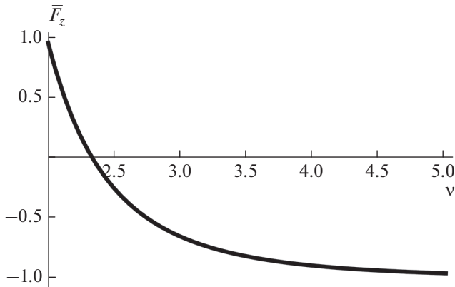
Рис. 2. Зависимость проекции плотности ponderомоторной силы взаимодействия решеток полуцилиндров.
