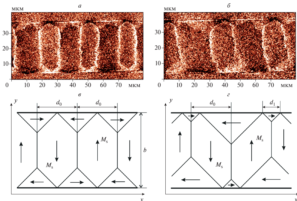
Рис. 2. Экспериментальное ( а, б ) и теоретическое ( в, з ) изменение формы магнитных доменов под действием внешнего магнитного поля для пленки составом FeNiCo 20 толщиной h = 15 нм, шириной b = 30 мкм и длиной l = 415 мкм. Внешнее магнитное поле H = 0 ( а, в ) и H = 5 Э ( б, з ).
