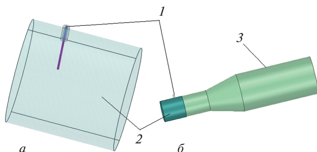
Рис. 2. Система передачи СВЧ-энергии от коаксиальной линии к резонаторной камере цилиндрического вида: переход с коаксиального входа на круглый волновод ( а ) и общий вид ( б ), где 1 – коаксиальный вход, 2 – волноводный тракт, 3 – цилиндрическая камера.
