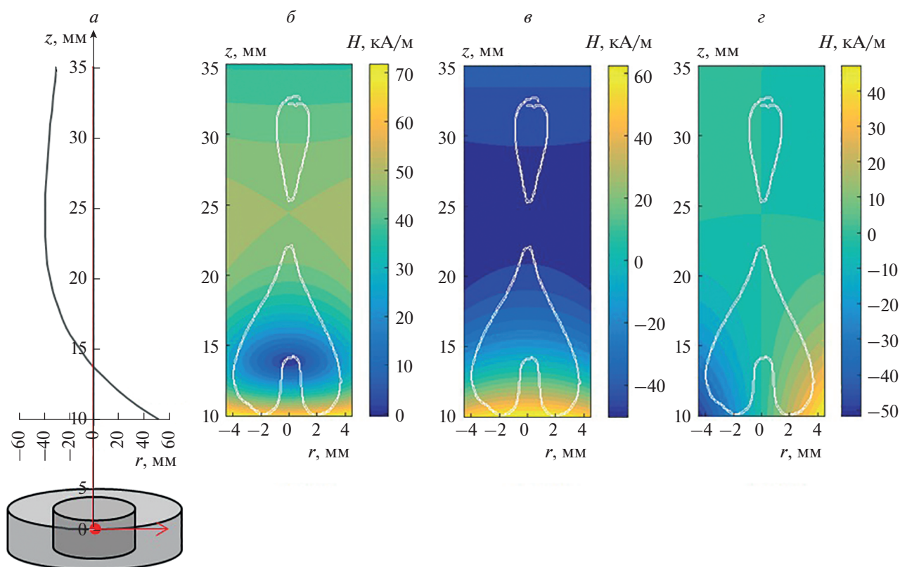
Рис. 4. Геометрия эксперимента (а), с расположением магнита, размеры которого представлены схематично, а также топология внешнего неоднородного магнитного поля в \text{kA/m} (его абсолютное значение (б), вертикальная (в) и радиальная (г) составляющие), совмещенная с изображением воздушной полости и пузырька в плоском канале, заполненном МЖ.
