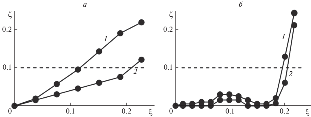
Рис. 3. Зависимости относительных изменений координат пика фокального пятна от относительных вариаций глубины волновода (а) и скорости звука (б). По оси абсцисс \xi = |\Delta H|/H_0 и \xi = |\Delta c|/c_0 ; по оси ординат: \zeta = |\Delta\tau_1|/\tau_1 (кривая 1) \zeta = |\Delta v_1|/v_1 (кривая 2).
