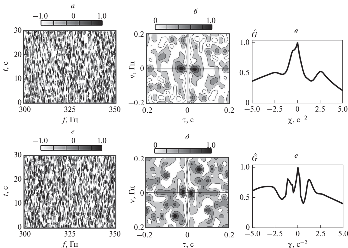
Рис. 1. Нормированные интерферограммы (а, с), голограммы (б, д) и функции обнаружения (е, е). Расстояния: 11.0 (а, б, е) и 11.5 км (с, д, е).
