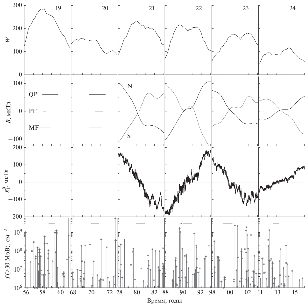
Рис. 1. Временные ряды сглаженных чисел Вольфа W и вертикальных компонент северного и южного полярного поля Солнца B_{N,S} , главного гауссового коэффициента магнитного поля Солнца g_{10} , и флюенсов F протонов с E > 30 МэВ в СПС в 19–24 циклах солнечной активности. Для 19–20 циклов показаны периоды инверсии по ранним наблюдениям полярного поля (MF), числа полярных факелов (PF) и положения волокон (QP) [7]. Найденные периоды понижения числа и флюенсов СПС во время инверсии поля показаны горизонтальными линиями на нижнем графике.
