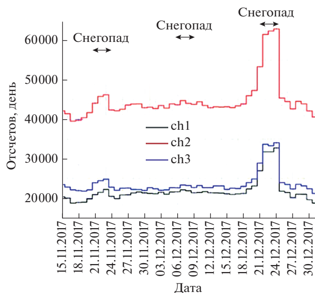
Рис. 1. Суточные графики “ch”-компоненты в эн-детекторах №№ 1, 2 и 3 в ангаре p -БНО в период 15.11.2017–30.12.2017.
