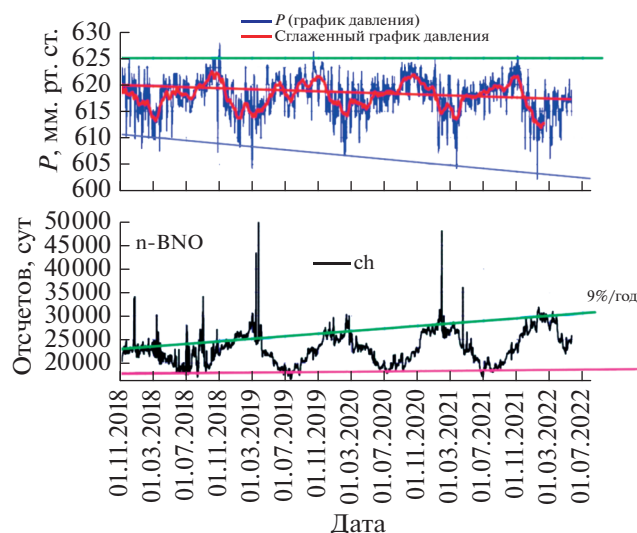
Рис. 2. Вариации давления (сверху) и “ch”-компоненты (снизу) на Баксане по данным детектора № 3 установки n-BNO с 2017 по 2022 гг.
