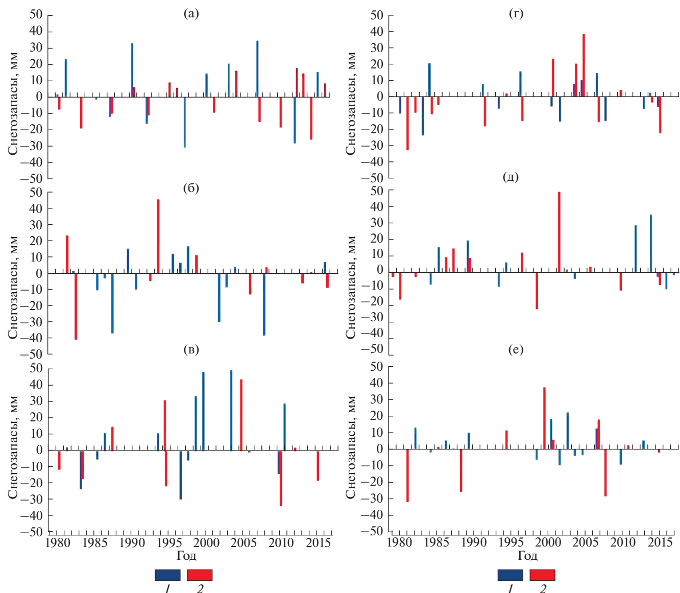
Рис. 1. Годы аномальных значений снеговзапасов. Реферные пункты: (а) – Калевала, (б) – Усть-Цильма, (в) – Вытегра, (г) – Опарино, (д) – Сухиничи, (е) – Порецкое. 1 – фактические данные (метеорологические станции), 2 – данные продукта GlobSnow (SWE).
