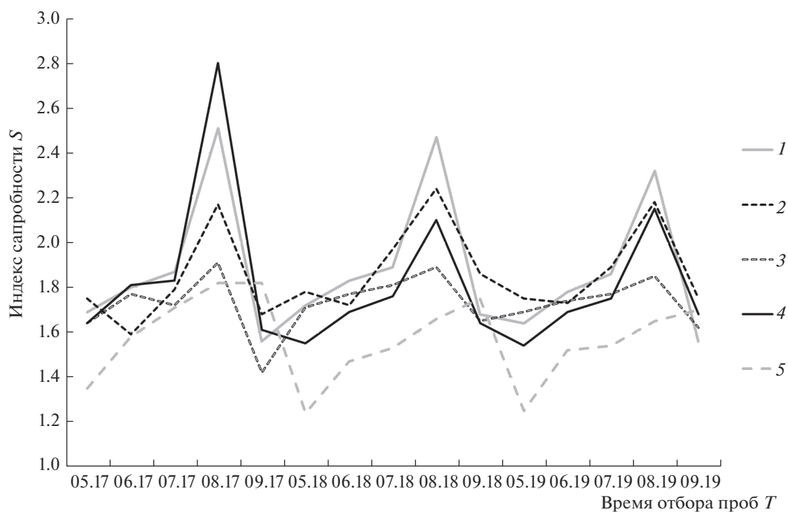
Рис. 3. Изменение численных значений индекса сапробности S в Иваньковском водохранилище в 2017–2019 гг. 1 – Шошинский плес; 2 – Верхневолжский плес; 3 – Средневолжский плес (с. Городня); 4 – Средневолжский плес (г. Конаково); 5 – Иваньковский плес.
