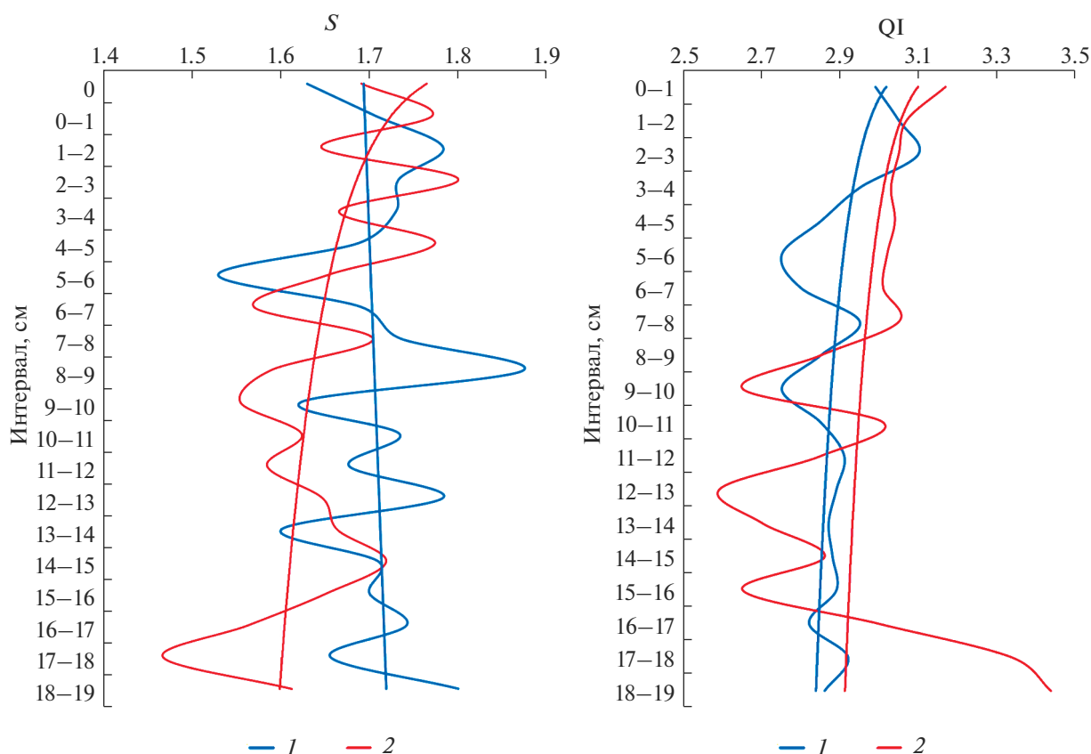
Рис. 8. Долговременные изменения численных значений S и QI в Ивановском водохранилище. Численные значения и результирующие линии: 1 – в районе Островов, 2 – в Перетрусовском заливе.
