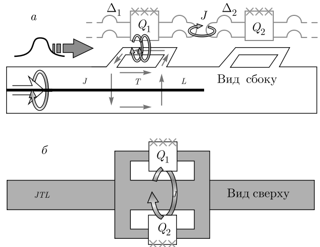
Рис. 2. Схема связанных джозефсоновских кубитов, управляемых униполярными импульсами: последовательное (а) и параллельное («симметричное») (б) расположение кубитов
