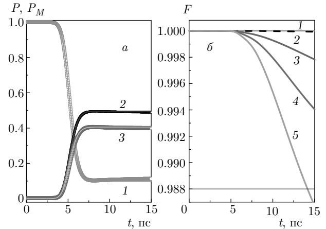
Рис. 6. (В цвете онлайн) а) Временная динамика населенностей двух связанных идентичных кубитов ( \Delta = \Delta_1 = \Delta_2 , J = 0.01 ГГц), где непрерывные кривые P(t) представляют результаты численного моделирования, а точками показаны аналитические решения P_M(t) . Здесь основному состоянию соответствуют красные кривые 1, промежуточному состоянию — черные кривые 2, возбужденному состоянию — синие кривые 3. б) Поведение «точности» F(t) для различных значений туннельных констант (красная кривая 1) соответствует \Delta = 0.0025 ГГц, черная 2 — \Delta = 0.01 ГГц, синяя 3 — \Delta = 0.05 ГГц, зеленая 4 — \Delta = 0.075 ГГц, оранжевая 5 — \Delta = 0.1 ГГц). Использованы следующие параметры импульса: \tau = 3 пс, t_0 = 1 пс, \varepsilon_m = 0.65 ГГц
