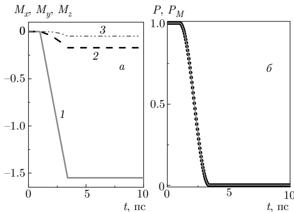
Рис. 4. (В цвете онлайн) а ) Динамика элементов матрицы вращения, где M_x представляет красная кривая 1, M_y — черная штриховая кривая 2, M_z — синяя штрихпунктирная кривая 3. б ) Временная эволюция населенности основного состояния кубита с туннельной энергией \Delta = 0.05 ГГц, где красная кривая — результат решения уравнения Шредингера P(t) , черные точки — аналитическое решение P_M(t) по Магнусу (39). Параметры управляющего прямоугольного импульса: \tau = t_{off} - t_{in} = 2.4 пс ( t_{in} = 1 пс и t_{off} = 3.4 пс), \varepsilon_m = 0.3 ГГц
