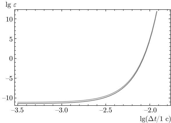
Рис. 2. Ограничение на параметр \varepsilon в зависимости от длительности начального нейтринного всплеска \Delta t (логарифмы десятичные) при M_\nu = 0.02 M_\odot . Нижняя кривая соответствует уровню шума T^* \approx 29 К, верхняя кривая — уровню возможного сигнала T^* \approx 135 К
