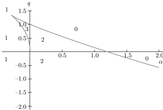
Рис. 1. Конфигурационное пространство метрики (4), разделенное на области с разным числом горизонтов, соответствующим приведенным на рисунке цифрам
