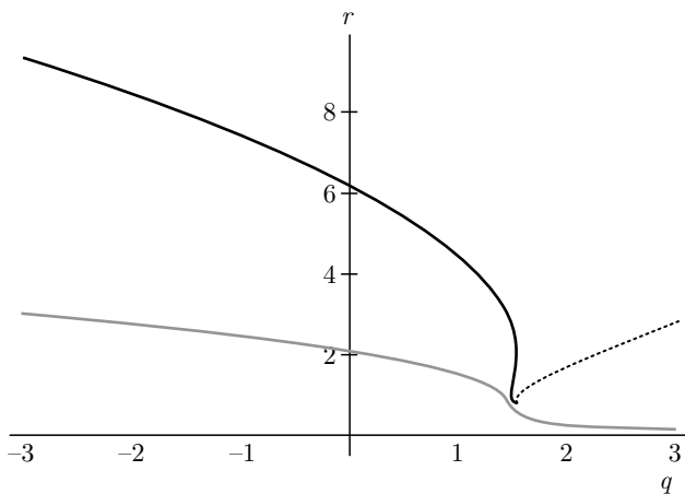
Рис. 7. Радиус последней устойчивой орбиты (верхняя кривая) для \alpha = -0.4 . Нижняя кривая соответствует радиусу горизонта событий. Пунктирная линия соответствует орбитам с нулевым угловым моментом
