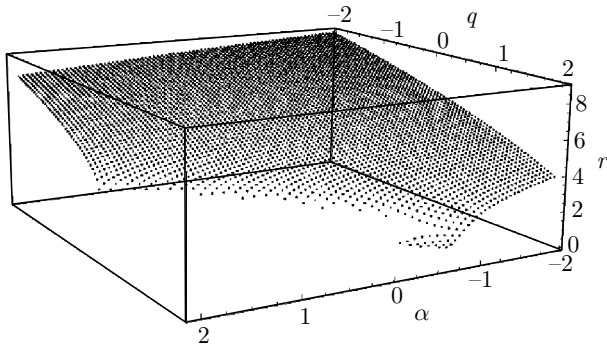
Рис. 6. Радиус последней устойчивой орбиты r(q, \alpha)
