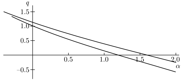
Рис. 4. Критические кривые, соответствующие конечному сдвигу радиуса горизонта и размера тени. Верхняя кривая — сдвиг размера тени, нижняя — сдвиг радиуса горизонта
