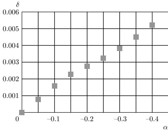
Рис. 5. Параметр отклонения \delta = |D(\alpha) - D(0)|/D(0) для черной дыры с тенью, соответствующей D_{sh} = 3\sqrt{3}
