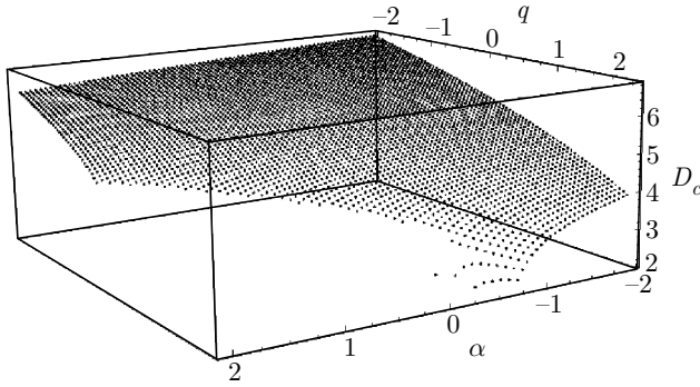
Рис. 3. Зависимость критического прицельного параметра D_c от q и \alpha
