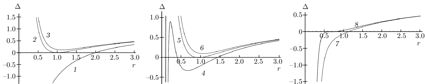
Рис. 2. Графики функции \Delta метрики (4) для различных значений q и \alpha : 1 — \alpha = 0, q = 0 ; решение Шварцшильда; 2 — \alpha = 0, q = 1 , решение Рейснера–Нордстрема с критическим зарядом; 3 — \alpha = 0, q = 9/8 , «голая сингулярность», описываемая метрикой Рейснера–Нордстрема; 4 — \alpha = -0.1, q = 0.89 , метрика (4) с тремя горизонтами; 5 — \alpha = -0.1, q = 1.1 , метрика (4) с двумя горизонтами; 6 — \alpha = -0.1, q = 1.2 , метрика (4) с одним компактным горизонтом; 7 — \alpha = -0.4, q = 1.33 , метрика (4) с одним горизонтом; 8 — \alpha = -0.296, q = 1.33 , конечная точка кривой исчезновения горизонта
