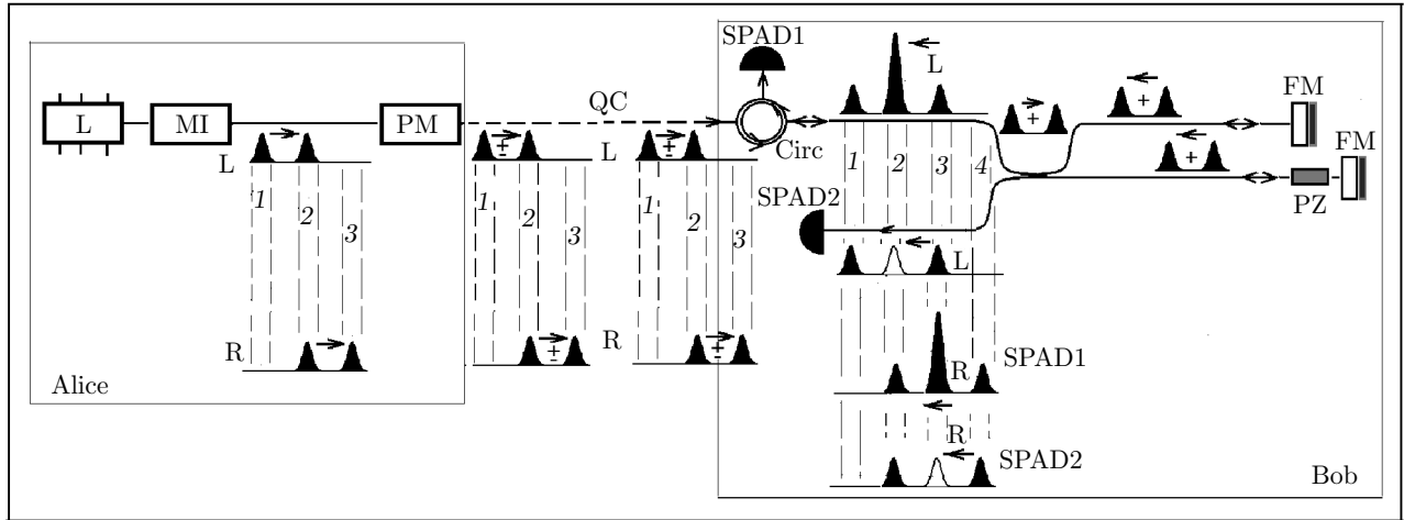
Рис. 1. Передающая сторона (Alice): L — лазер, работающий в CW-моду, MI — модулятор интенсивности, PM — фазовый модулятор. Весь оптический тракт на передающей станции выполнен на волокне, сохраняющем поляризацию. Приемная часть (Bob): весь оптический тракт выполнен на стандартном одномодовом SM-волокне. Circ — волоконный поляризационно независимый циркулятор. SPAD1,2 — однофотонные лавинные детекторы. FM — фарадеевское зеркало. PZ — управляемый пьезоэлемент для выравнивания разности хода в верхнем и нижнем плечах интерферометра. QC — линия связи на основе SM-волокна. Стрелками показана эволюция состояний
