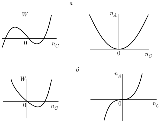
Рис. 2. Графики потенциальной энергии W(n_C) и функции n_A(n_C) при n_{A0} = n_{BC0} = 3 , n_{C0} = n_{AB0} = 2 , n_0 = 1 ; \Omega_2/\Omega_1 — четное (а), нечетное (б)
