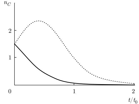
Рис. 4. Временные зависимости плотности атомов типа C при \alpha = 1/2 (пунктирная линия), 2 (сплошная линия)
