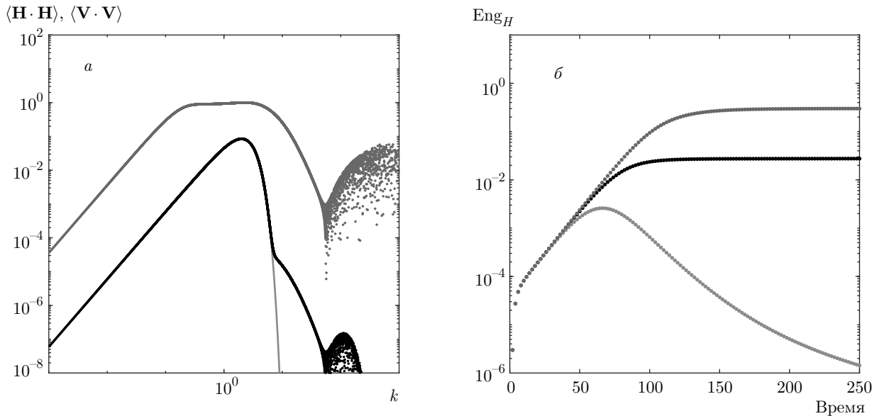
Рис. 3. (В цвете онлайн) Динамический спектр. а) Энергетические спектры магнитной (синие точки) и кинетической (черные точки) энергий, красная линия соответствует начальному гауссову кинетическому спектру. б) Зависимости полной магнитной энергии от времени (синяя линия — сохранение суммарной энергии и формы спектра, черная — добавка магнитного поля к гауссову спектру, красная — постоянная подкачка магнитной энергии с сохранением суммарной энергии равной 1
