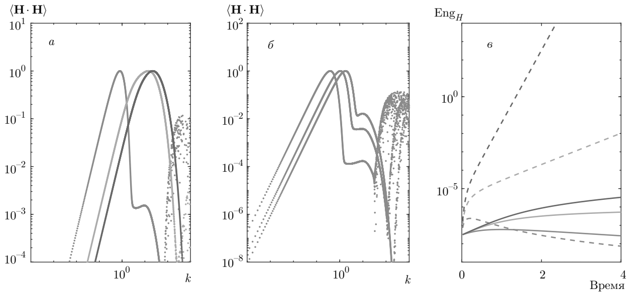
Рис. 1. (В цвете онлайн) Гауссов спектр. а) Энергетические спектры магнитной энергии. б) Спектры энергии в докритическом режиме для трех моментов времени t = 0.25, 2.5, 25 (сверху вниз соответственно). в) Изменение суммарной магнитной энергии со временем для трех режимов: докритического Rm = 50 (красный), критического Rm = 250 (зеленый), сверхкритического Rm = 1000 (синий). Сплошные линии на рис. в) соответствуют стандартному гауссову спектру, штриховые — спектру, сдвинутому на малые масштабы. Точки на рис. а) , выпадающие из спектральных кривых, — артефакт численного преобразования Фурье на неравномерной сетке, они могут быть немного отодвинуты путем измельчения сеточного шага, но избавиться от них совсем невозможно, поэтому мы их оставили здесь и на других рисунках, чтобы не вносить внешние исправления в полученные результаты и показать ограничения выбранной численной реализации и разрешения
