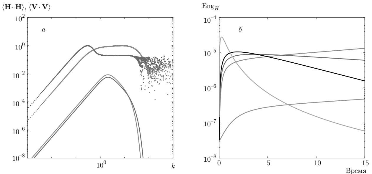
Рис. 2. (В цвете онлайн) Колмогоровский спектр. а) Энергетические спектры магнитной (точки) и кинетической (сплошные линии) энергий. б) Изменение суммарной магнитной энергии со временем для инерционных интервалов различной ширины k_{min} = 2, k_{max} = 2, 15, 20, 25, 100 , которые соответствуют зеленому, красному, синему, черному, голубому цветам. Для первых двух значений параметров наблюдается рост магнитной энергии, для оставшихся — затухание
